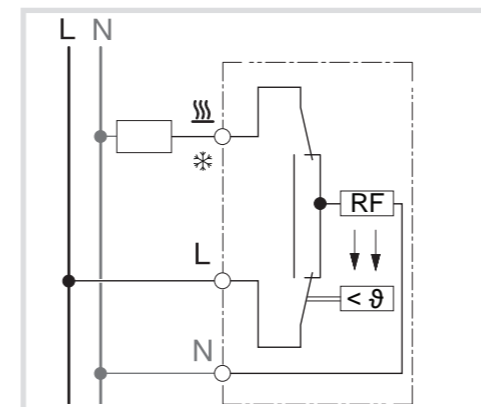
Figura 4: Collegamenti elettrici
