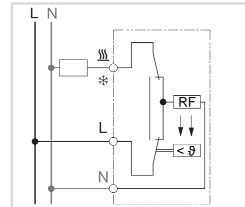
Afb. 4: Elektrische aansluiting
