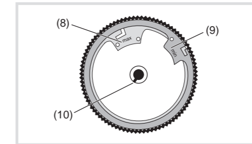
Afb. 5: Regelknop achteraanzicht
