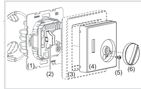
Afb. 1: Opbouw van het apparaat
