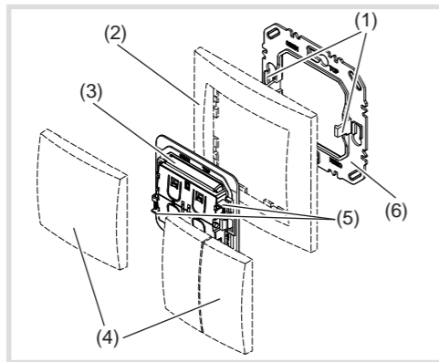
Bild 1: Geräteaufbau Wandsender
