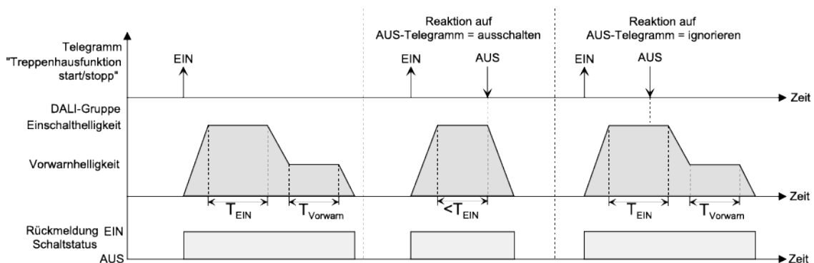
Bild 52: Ausschaltverhalten der Treppenhausfunktion mit Soft-Funktionen (als Beispiel mit Minimalhelligkeit = 0%)
