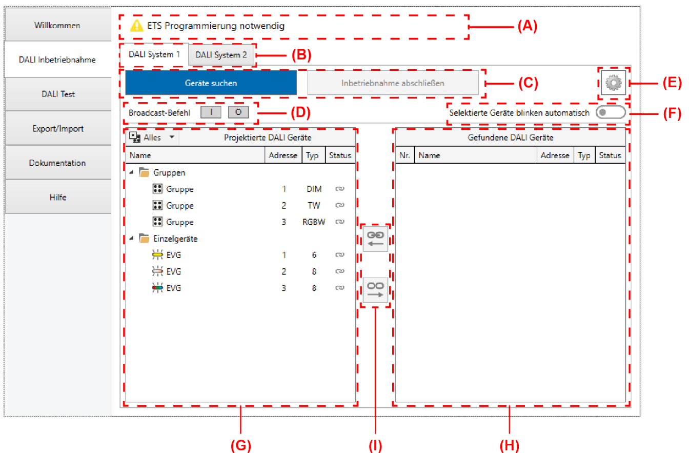
Bild 61: DALI-Inbetriebnahmeumgebung in der DCA
