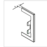
Wandanschlussblende Stahlblech
