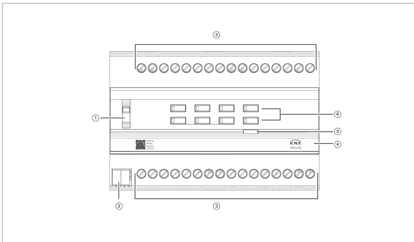
Bild 2: Geräteaufbau Schalt-/Jalousieaktor 16-/8fach
