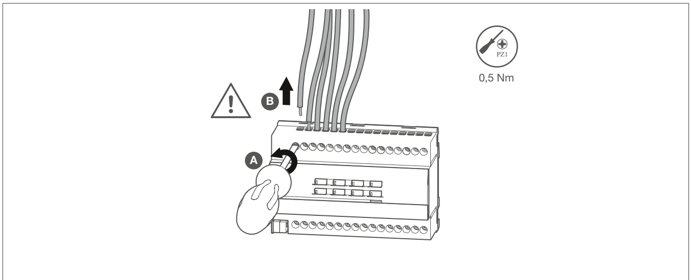
Bild 13: Lastleitungen abklemmen
