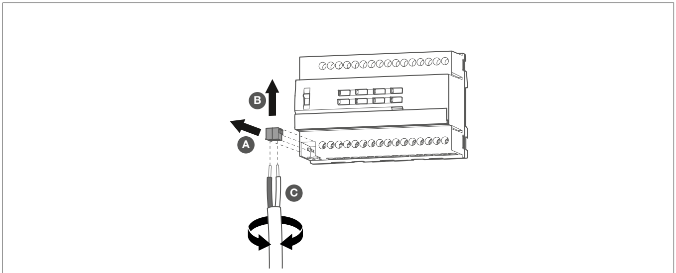
Bild 14: Busanschlussklemme abziehen
