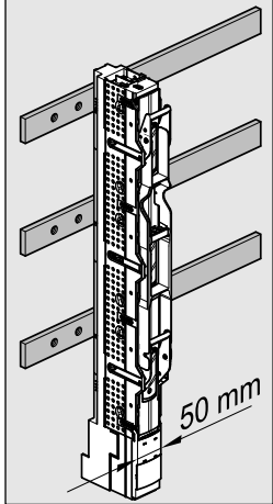
NH00 / 185 mm
