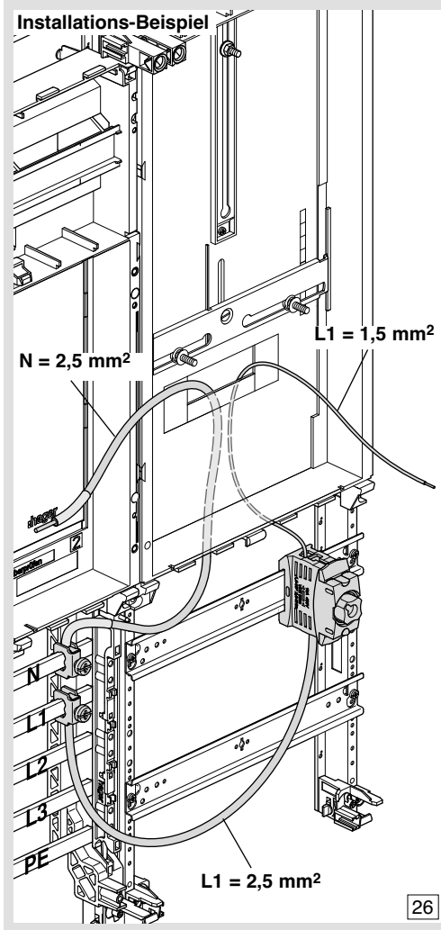
Installations-Beispiel
