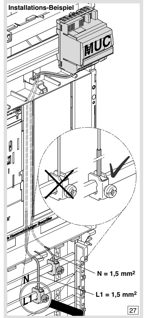
Installations-Beispiel
