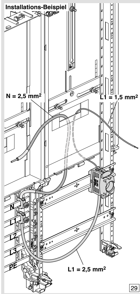
Installations-Beispiel
