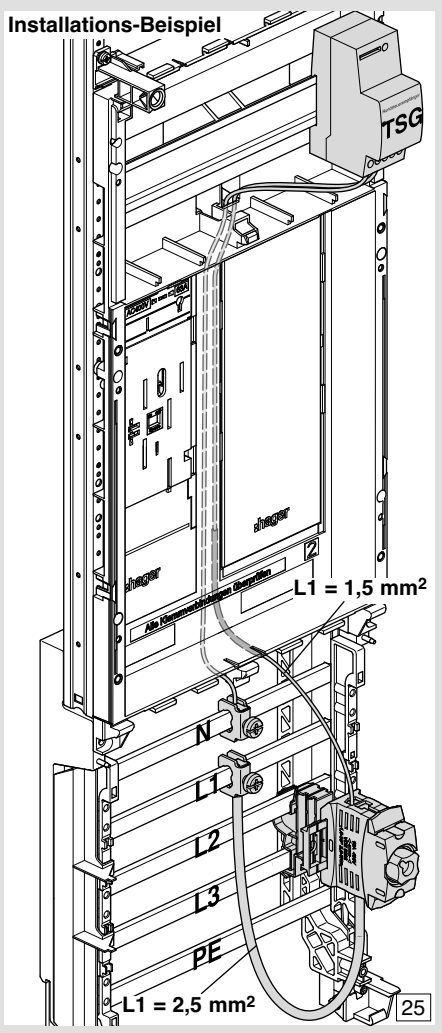
Installations-Beispiel
