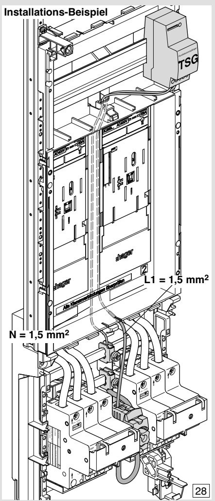
Installations-Beispiel
