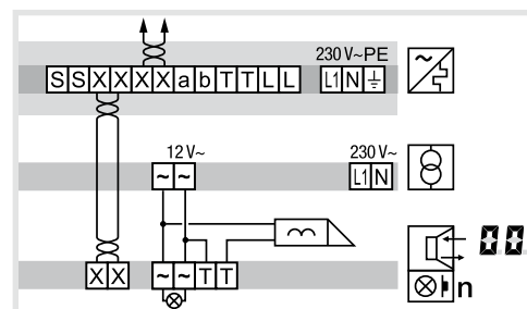
Afb. 7: Aansluiting deuropener op het deurstation
