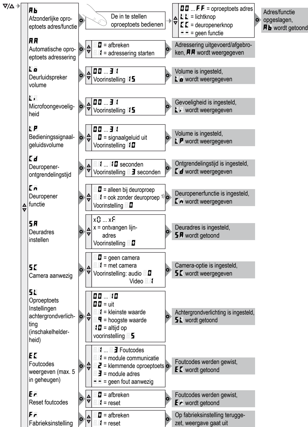
Afb. 9: overzicht systeeminstellingen
