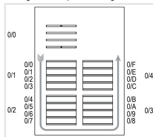
Afb. 10: Module-adres en automatische adressering oproep-toetsen
