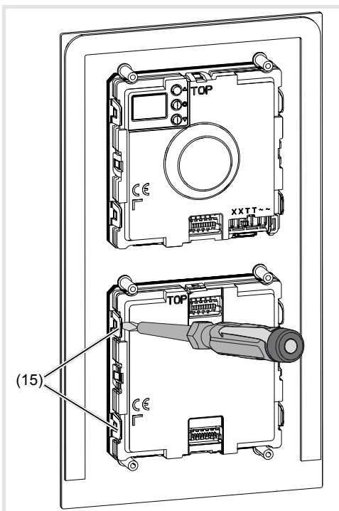
Afb. 13: Module ontgrendelen
