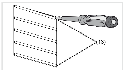
Afb. 11: Afnemen van de afdekstroken (13) Afdekstroken
