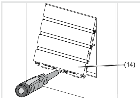
Afb. 12: Demontage opzetstuk oproepmodule (14) Opzetstuk oproepmodule
