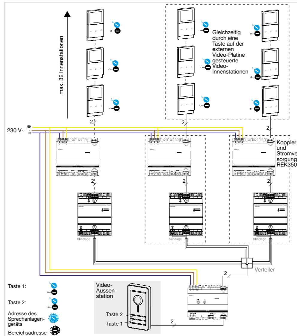
Abbildung 2: Funktionsschaltbild
