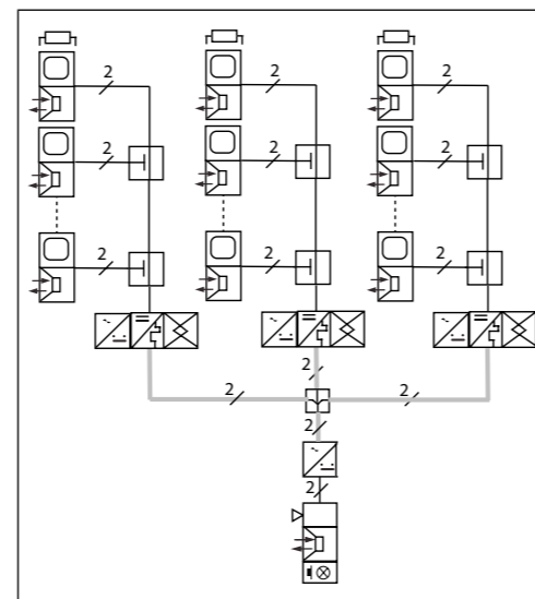
Abbildung 3: Anschlussbeispiel
