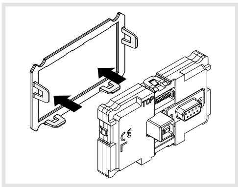
Bild 3: Montage der Halterung
