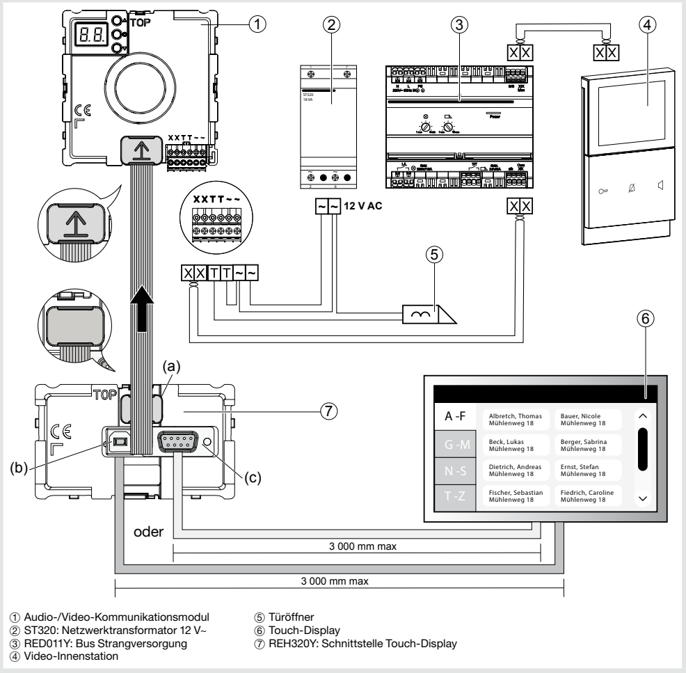
Bild 1: Geräteaufbau
