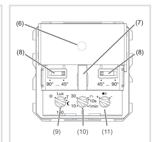
Image 8 : éléments de commande et de réglage
