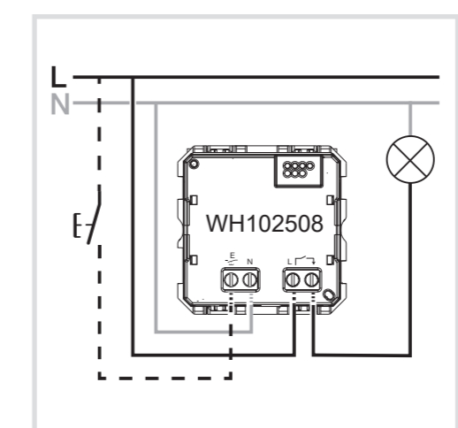
Image 6 : raccord du détecteur de mouvement tri filaire
