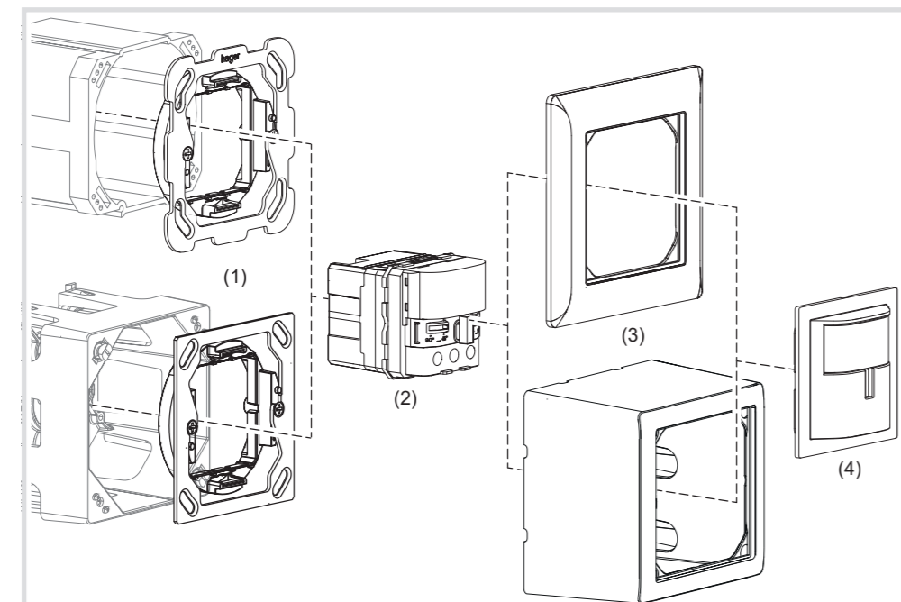
Image 1 : Description de l'appareil
