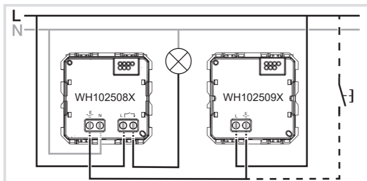
Image 7 : raccordement avec détecteur de mouvement trifilaire et poussoir de poste auxiliaire optionnel
