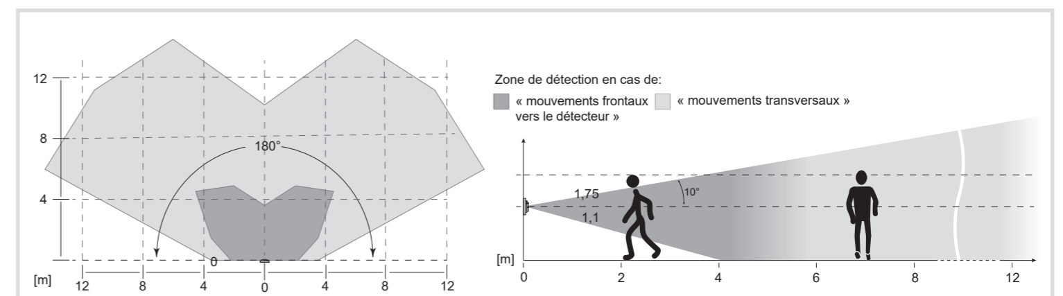
Image 5 : zone de détection du détecteur de mouvement pour une hauteur de montage nominale d'1,1 m
