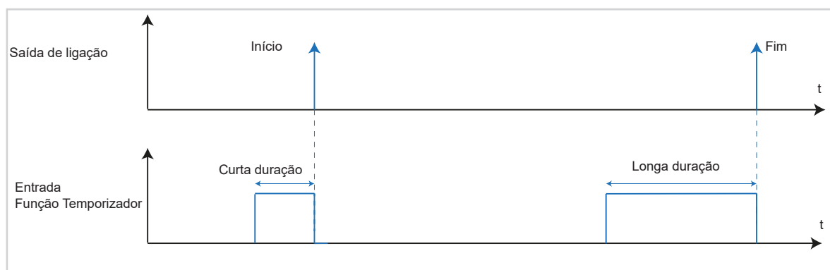
Figura 24: Diagrama de sinal e tempo Temporizador
