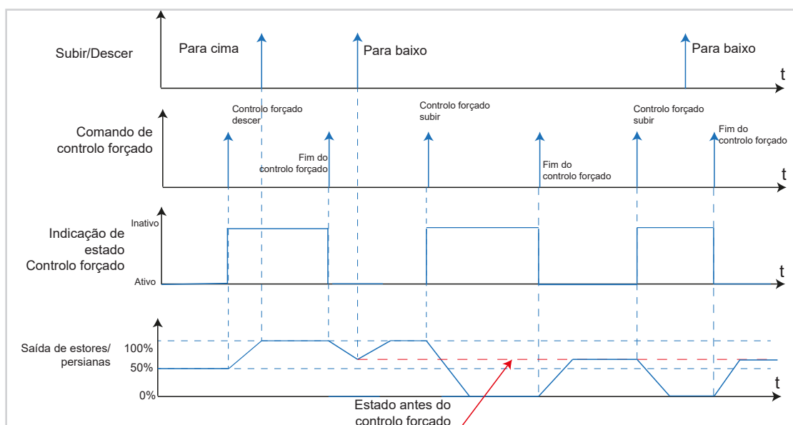
Figura 56: Diagrama de sinal e tempo Controlo forçado estore/persiana
