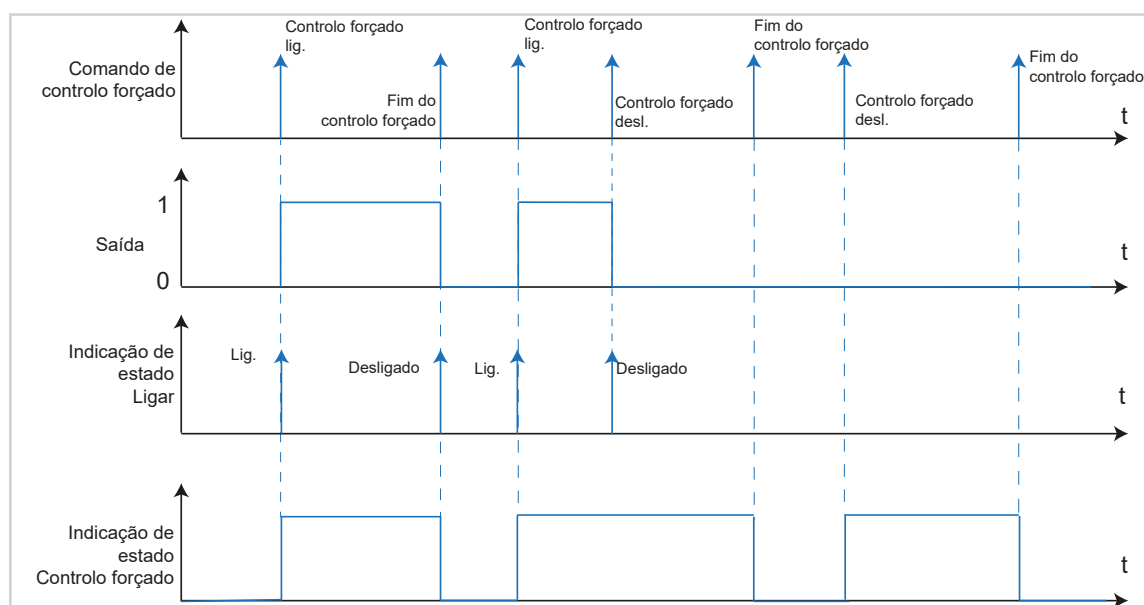
Figura 27: Diagrama de sinal e tempo Controlo forçado
