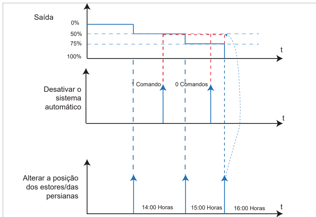
Figura 58: Diagrama de sinal e tempo Desativar o sistema automático
