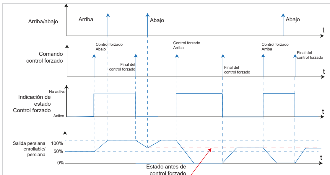
Figura 55: Gráfico señal-tiempo de Control forzado Persiana enrollable/Persiana
