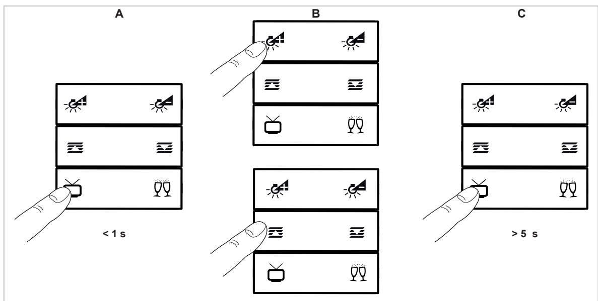
Figura 29: Activación de escena
