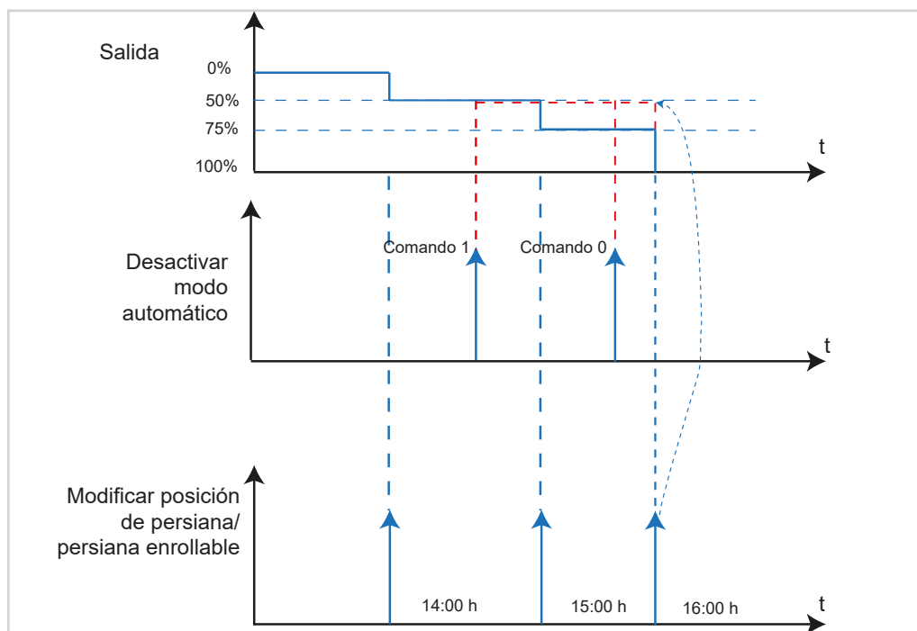
Figura 57: Gráfico señal-tiempo Desactivar modo automático
