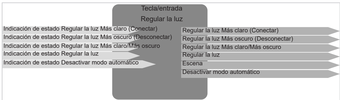
Figura 5: Señales de entrada/salida Función Regular la luz
