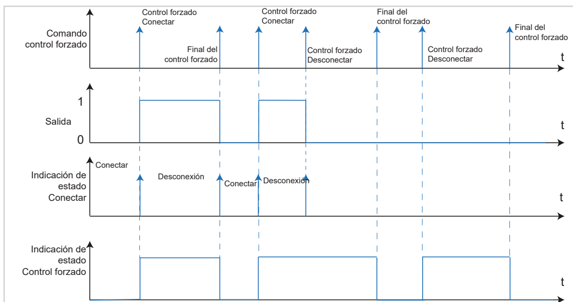
Figura 26: Gráfico señal-tiempo de control forzado
