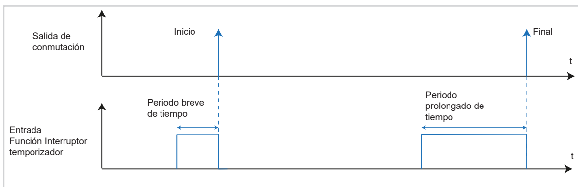
Figura 23: Gráfico señal-tiempo interruptor temporizador
