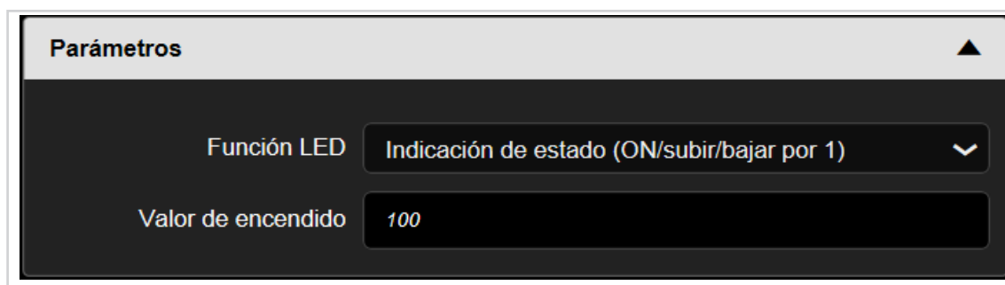
Figura 35: Fijar el valor de regulación de luz
