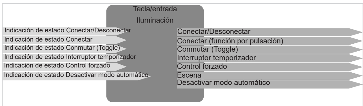
Figura 4: Señales de entrada/salida Función Iluminación
