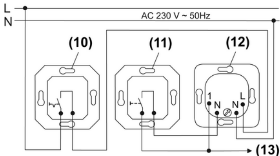
Afbeelding 4: Aansluitvoorbeeld kleuromschakeling via nulleider
