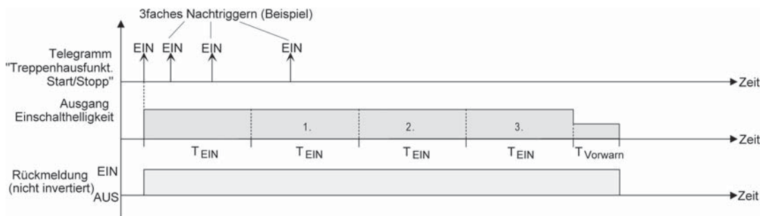
Bild 28: Zeitverlängerung der Treppenhausfunktion
