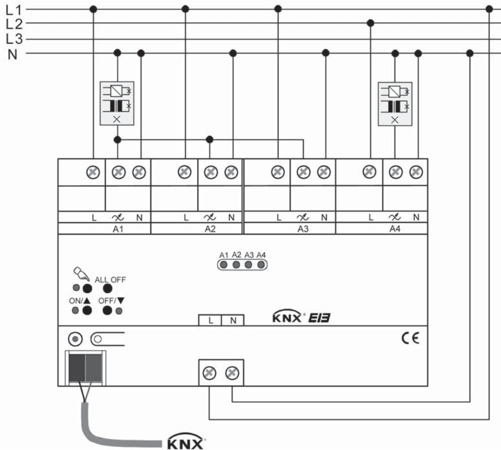
Bild 5: Elektrischer Anschluss bei Parallelverdrahtung von Ausgängen (Beispiel)
