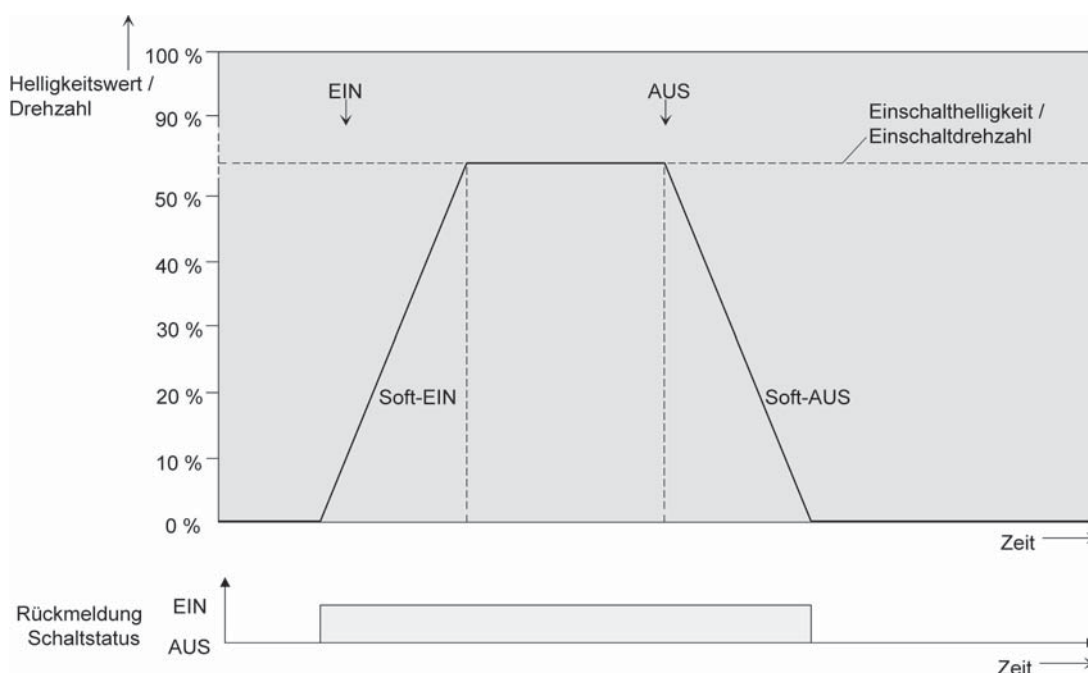
Bild 15: Dimmverhalten der Soft-EIN/AUS-Funktionen (als Beispiel)
