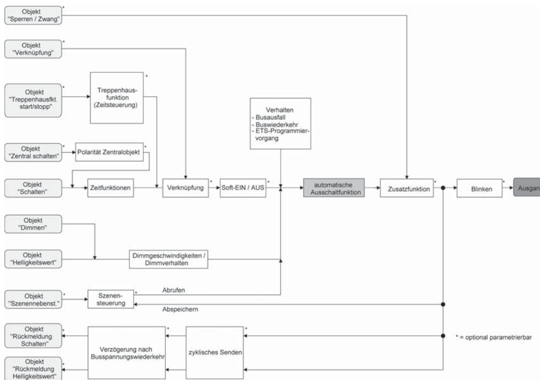
Bild 18: Funktionsschaltbild der automatischen Ausschaltfunktion
