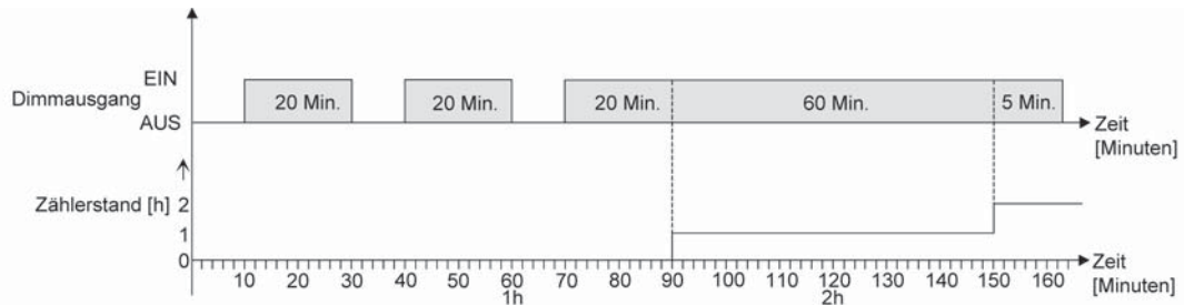
Bild 30: Funktionsweise des Betriebsstundenzählers (am Beispiel eines Vorwärtszählers)
