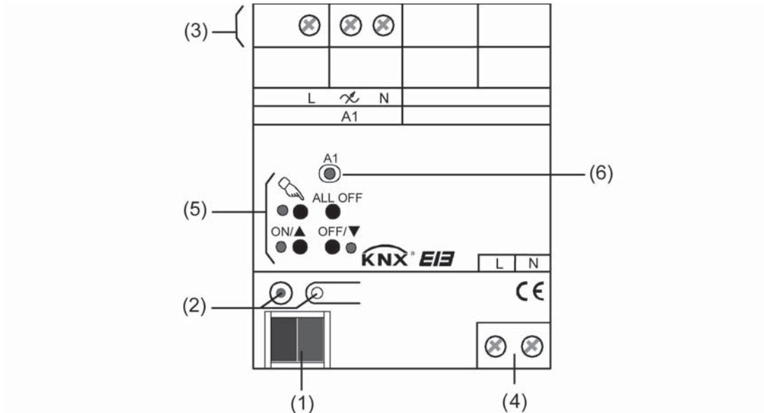
Bild 1: Aufbau der Gerätevariante 1fach
