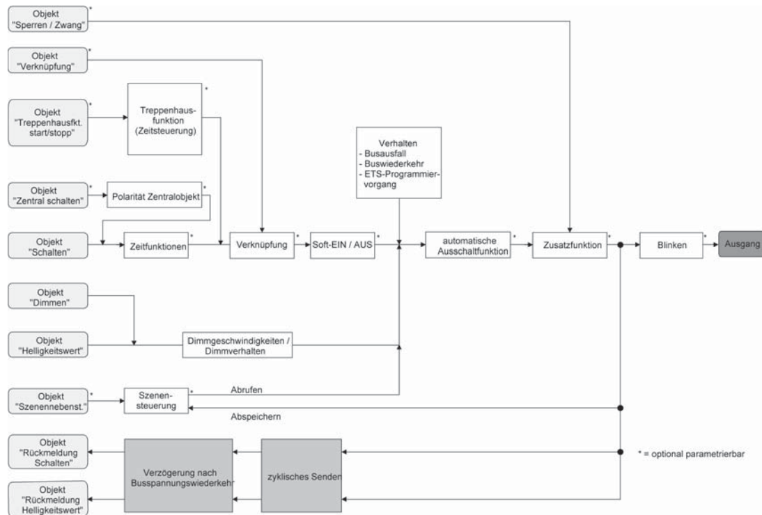
Bild 13: Funktionsschaltbild der Rückmeldungen
