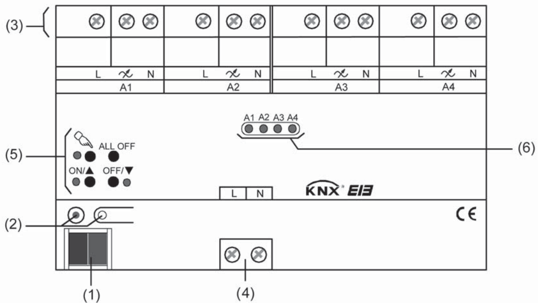
Bild 3: Aufbau der Gerätevariante 4fach
