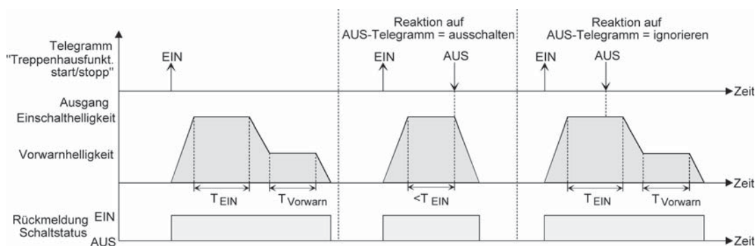
Bild 23: Ausschaltverhalten der Treppenhausfunktion mit Soft-Funktionen (als Beispiel mit Minimalhelligkeit = 0 %)
