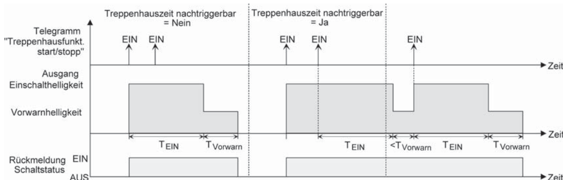
Bild 20: Einschaltverhalten der Treppenhausfunktion ohne Soft-Funktionen
