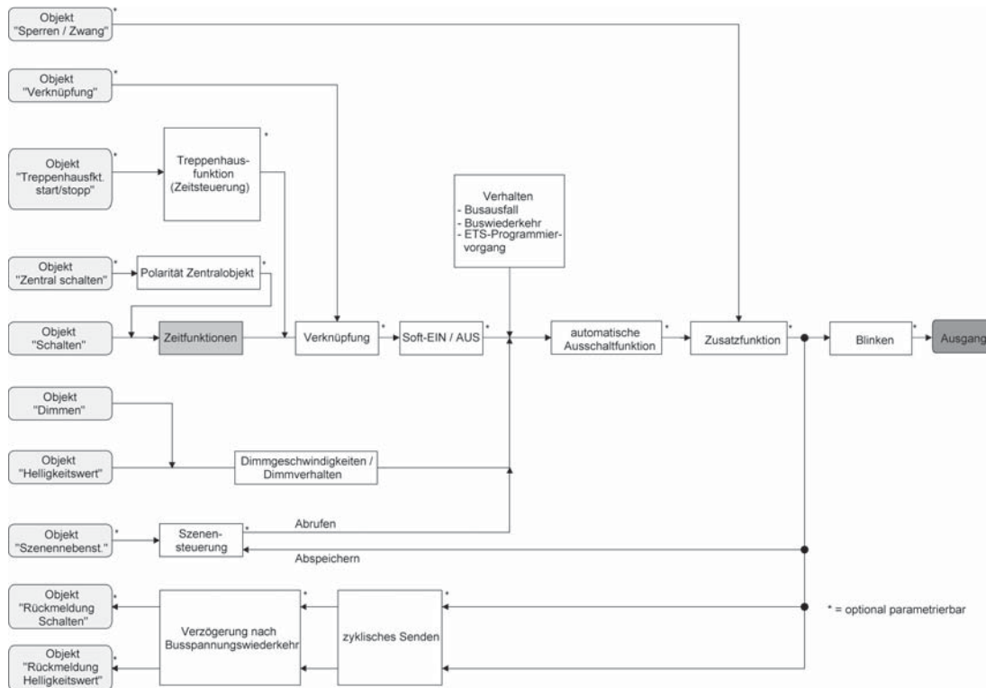
Bild 14: Funktionsschaltbild der Zeitfunktionen
