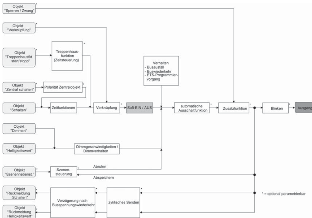
Bild 16: Funktionsschaltbild der Soft-Funktionen
