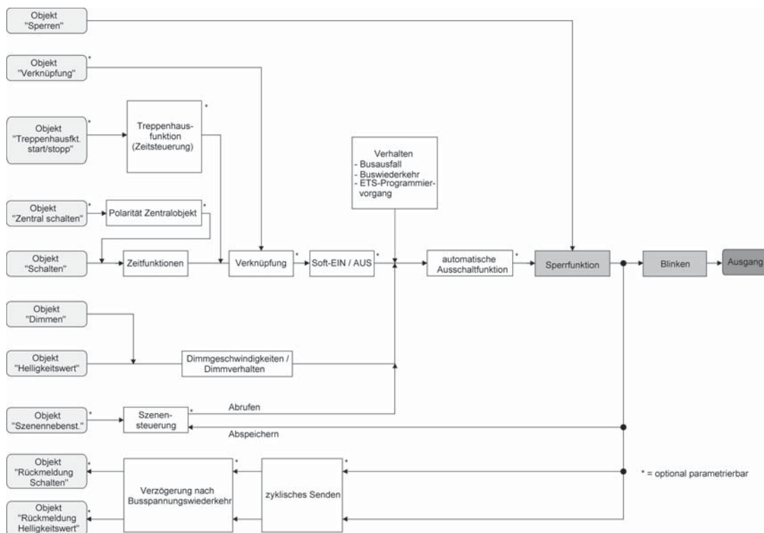
Bild 31: Funktionsschaltbild der Sperrfunktion
