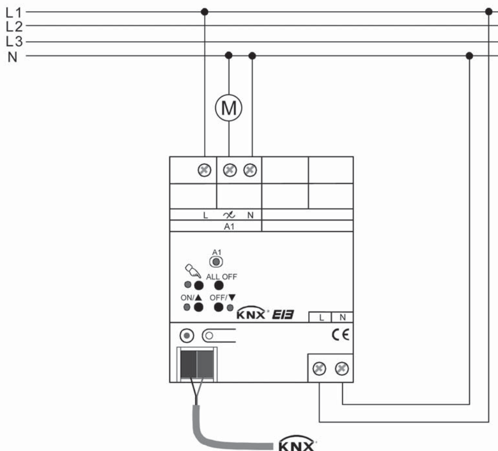
Bild 6: Elektrischer Anschluss von Einphasen-Elektromotoren
