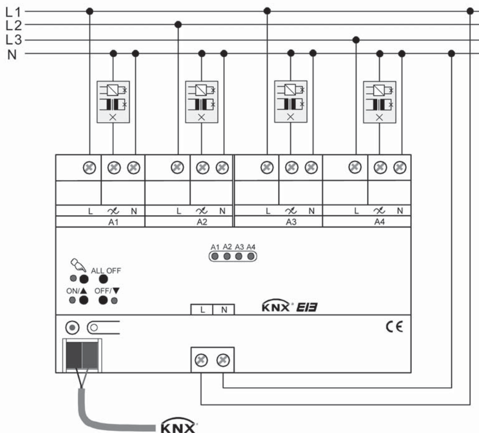
Bild 4: Elektrischer Anschluss (am Beispiel der Gerätevariante 4fach)
