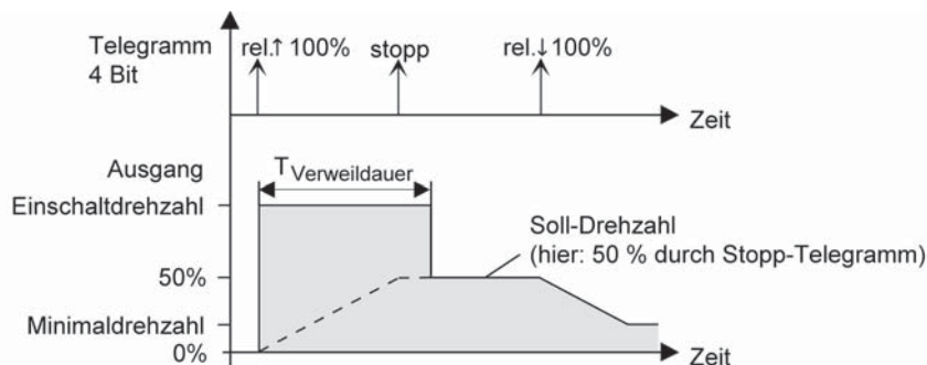
Bild 41: Einschalt Drehzahl und Soll-Drehzahl bei relativen Dimmbefehlen
