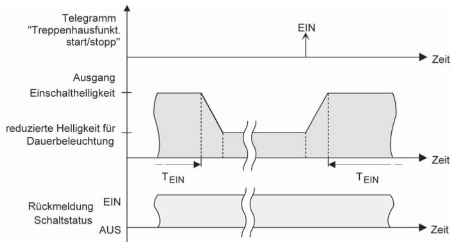
Bild 27: Die Dauerbeleuchtung der Treppenhausfunktion mit Soft-AUS-Funktion
