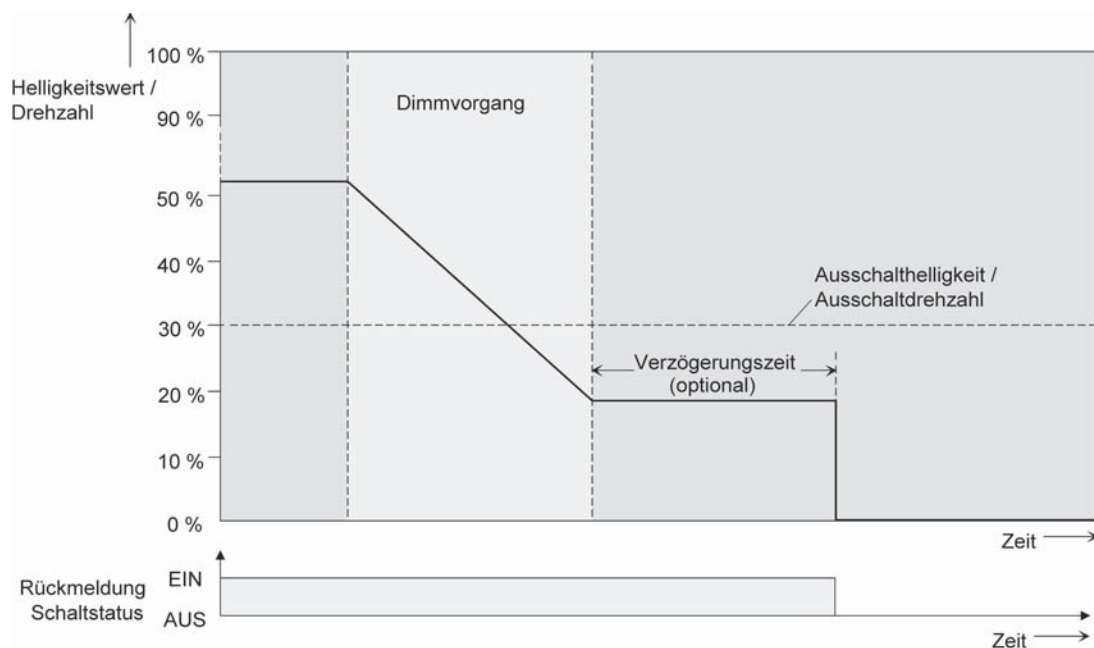
Bild 17: Dimm- und Schaltverhalten der automatischen Ausschaltfunktion
