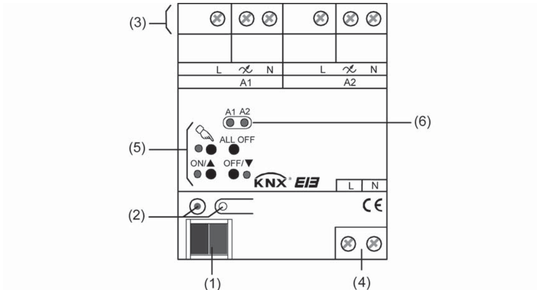
Bild 2: Aufbau der Gerätevariante 2fach
