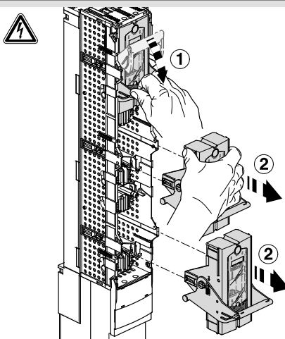
Montageart 2; Montage unter Spannung Kind of assembly 2; Assembly under voltage
