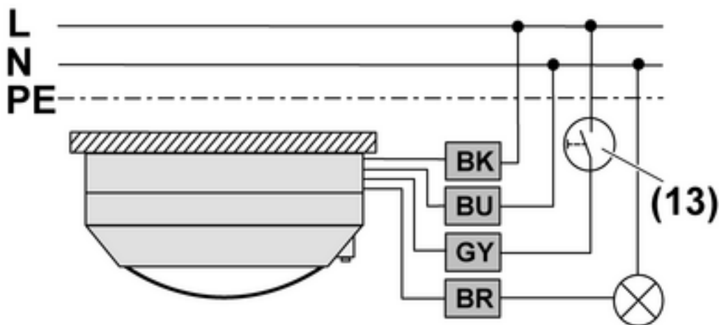
Afbeelding 6: Aansluitschema
