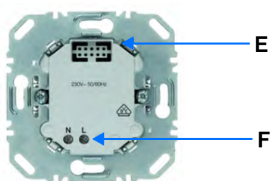
Voeding 230V~
