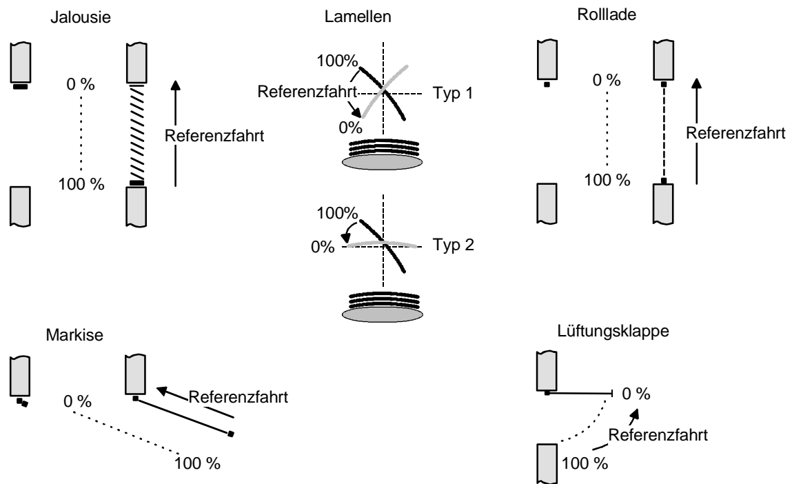
Bild 29: Referenzfahrt
