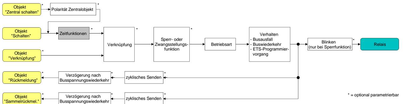
Bild 13: Funktionsschaltbild der Zeitverzögerungen
