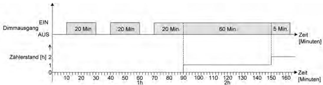
Bild 32: Funktionsweise des Betriebsstundenzählers (am Beispiel eines Vorwärtszählers)
