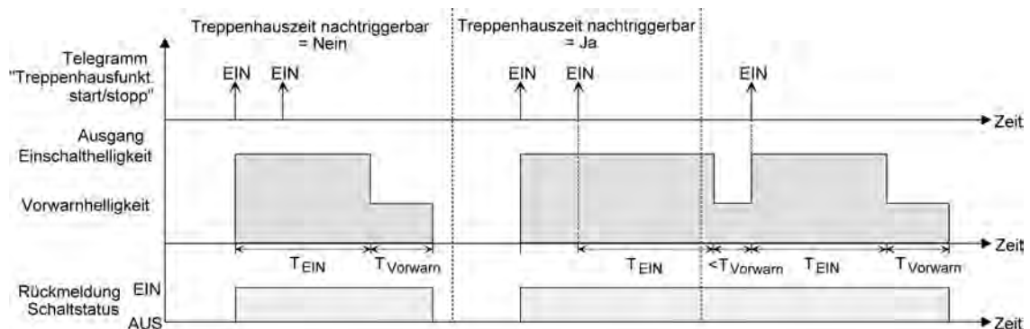
Bild 22: Einschaltverhalten der Treppenhausfunktion ohne Soft-Funktionen
