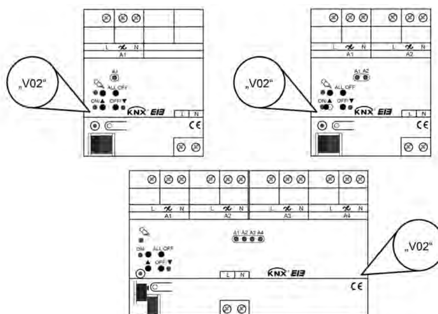
Bild 9: Position der Kennzeichnung der Gerätegeneration
