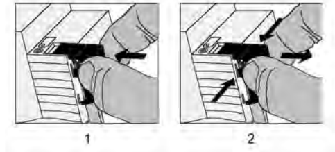
Bild 7: Abdeckkappe für Busanschluss anbringen / entfernen
