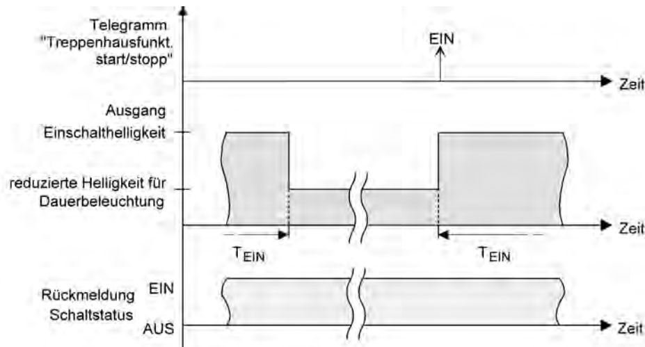
Bild 28: Die Dauerbeleuchtung der Treppenhausfunktion ohne Soft-Funktionen
