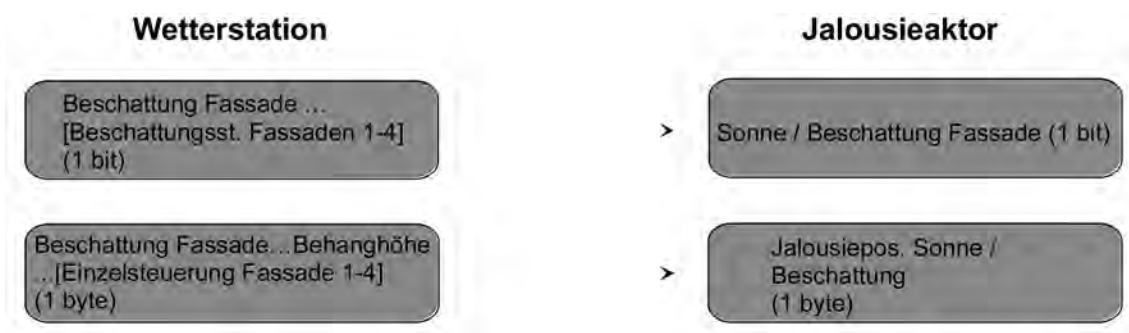
Bild 29: Projektierung der Kommunikationsobjekte für Anwendungsbeispiel V.
