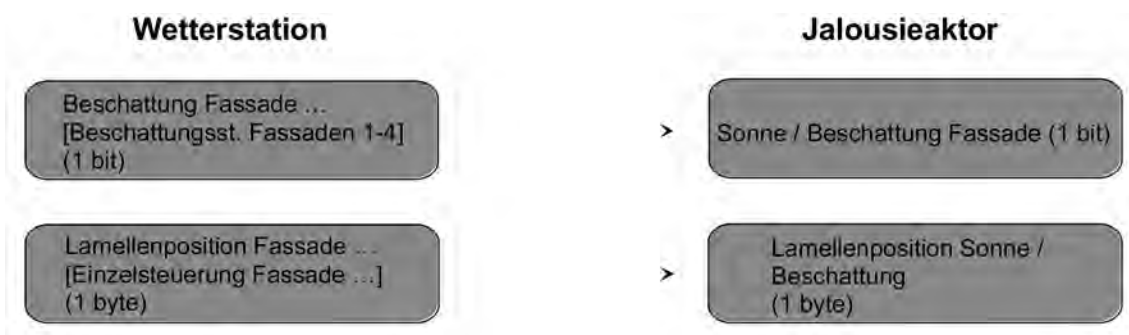
Bild 27: Projektierung der Kommunikationsobjekte für Anwendungsbeispiel III.
