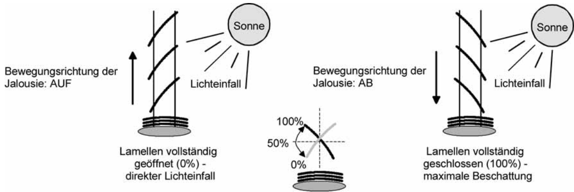
Bild 30: Typ 1 - Lamellenjalousien mit schräger Lamellenstellung in beide Fahrrichtungen
