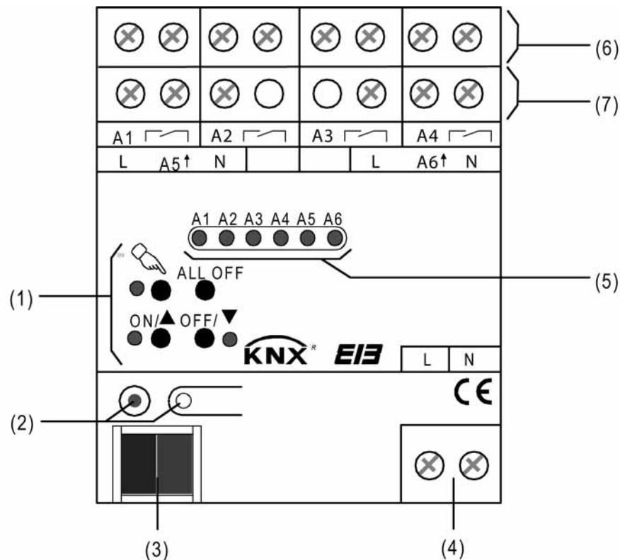
Bild 1: Geräteaufbau
