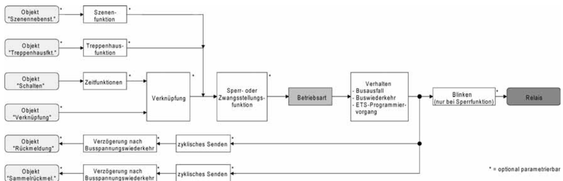
Bild 14: Funktionsschaltbild "Betriebsart"
