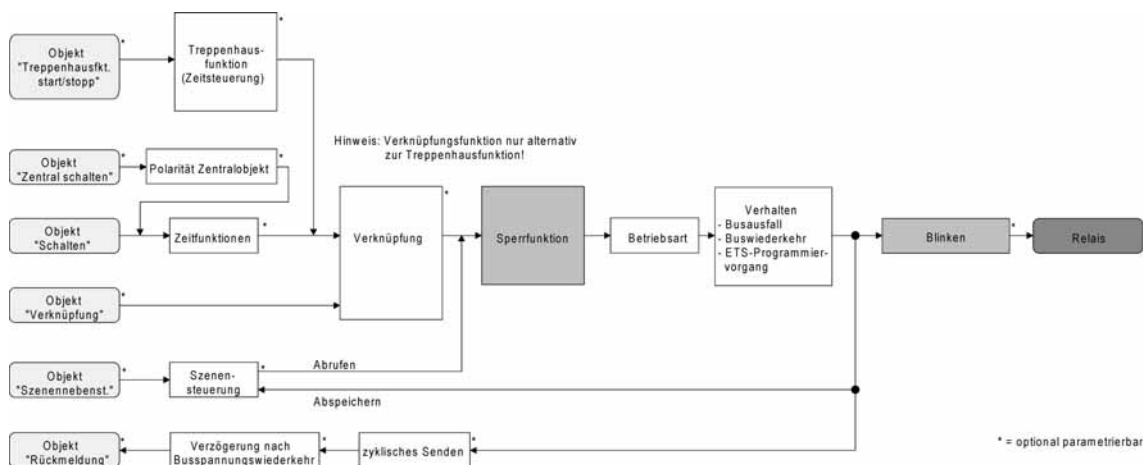
Bild 24: Funktionsschaltbild der Sperrfunktion
