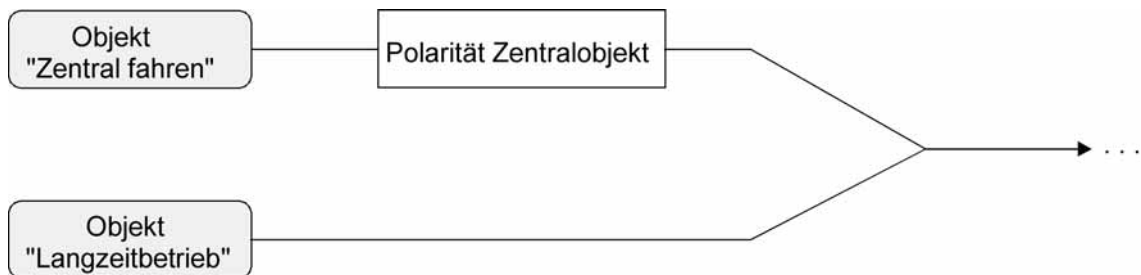
Bild 12: Funktionsschaltbild "Zentral fahren"
