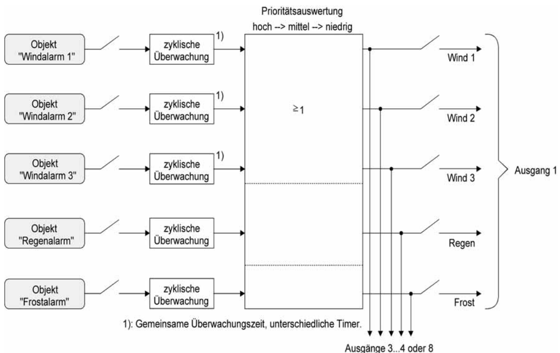
Bild 13: Funktionsschaltbild der Sicherheitsfunktionen
