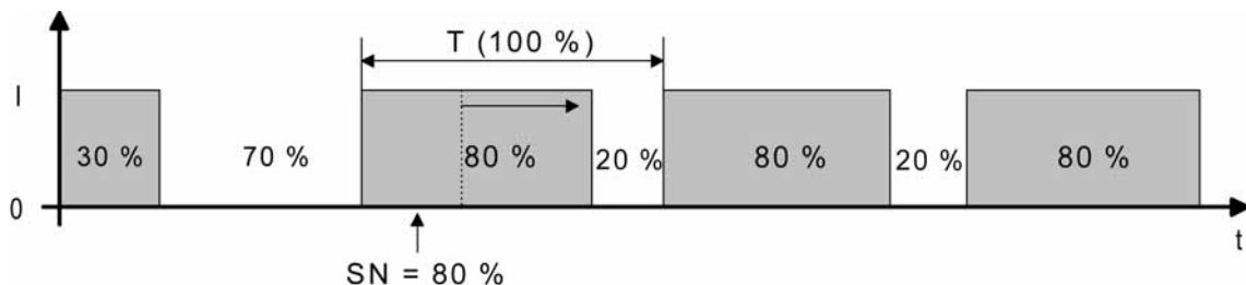
Bild 62: Stellgrößenänderung z. B. von 30 % auf 80 % während Öffnungsphase des Ventils
