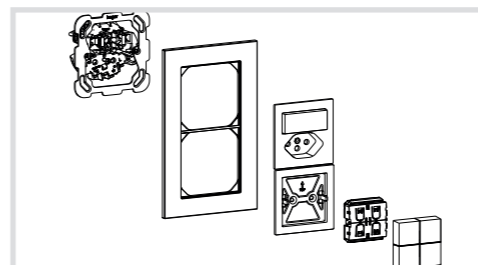
Image 6 : Montage dans l'installation existante
