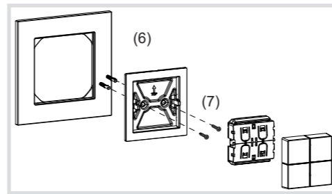
Image 4 : Montage avec des vis
