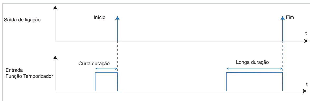
Figura 29: Diagrama de sinal e tempo Temporizador
