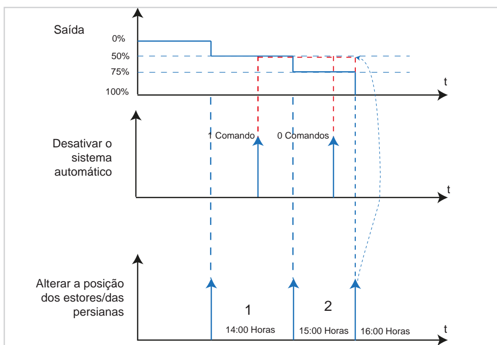
Figura 68: Diagrama de sinal e tempo Desativar o sistema automático
