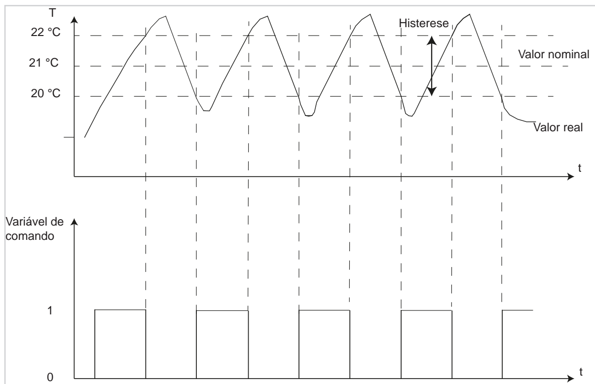
Figura 18: Regulação de 2 pontos
