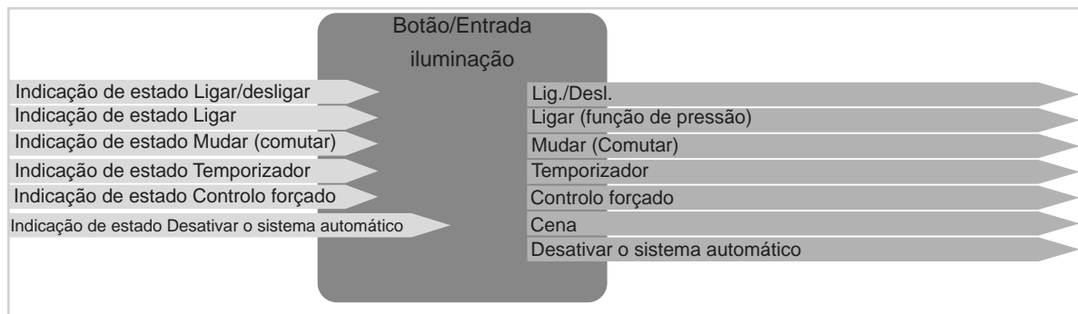
Figura 6: Sinais de entrada/saída Função iluminação
