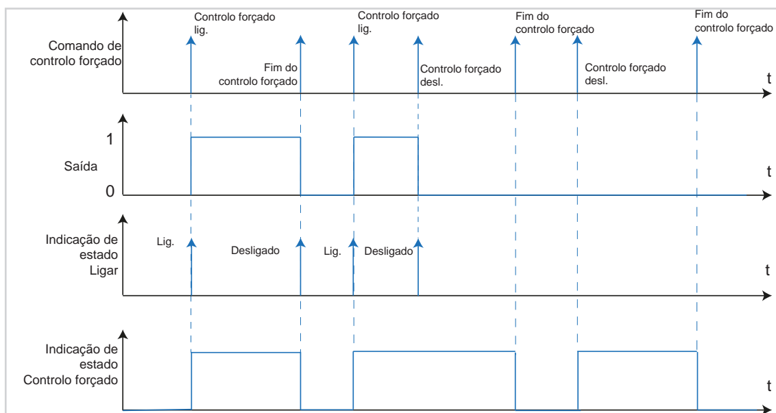
Figura 32: Diagrama de sinal e tempo Controlo forçado
