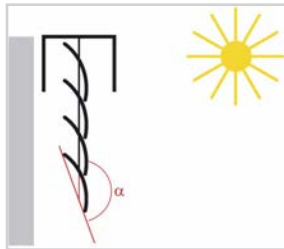
Figura 47: Posição da persiana Posição final inferior 100 %
