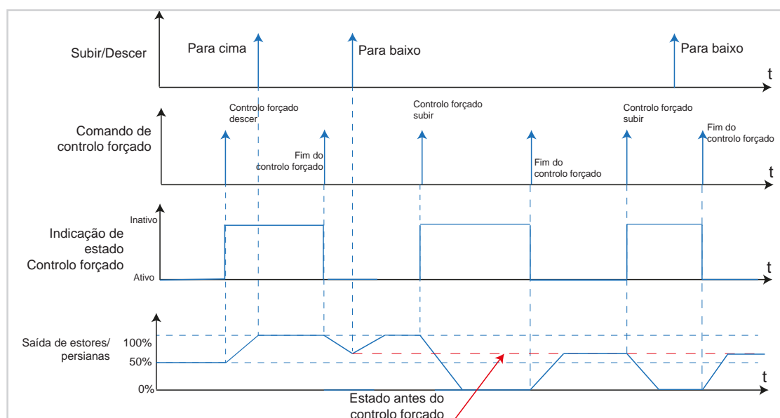
Figura 66: Diagrama de sinal e tempo Controlo forçado estore/persiana
