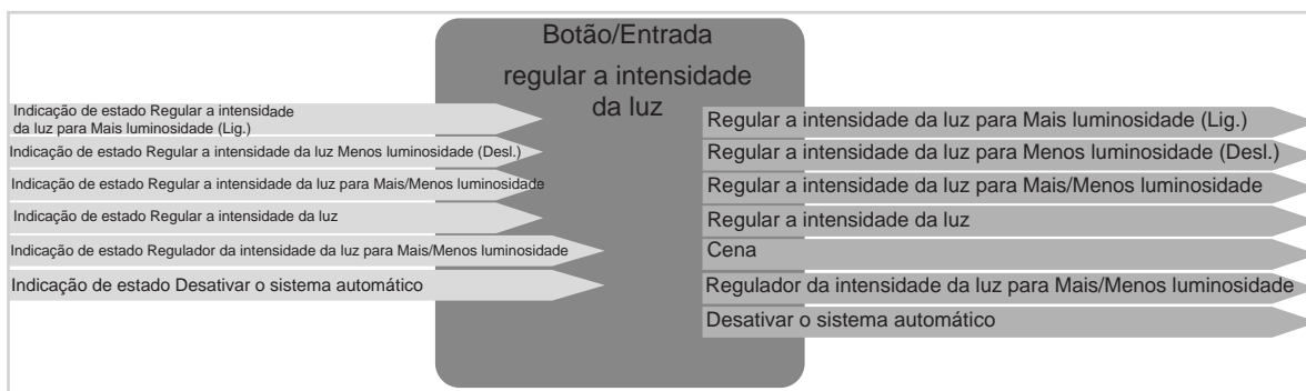
Figura 7: Sinais de entrada/saída Função de regulação da intensidade da luz
