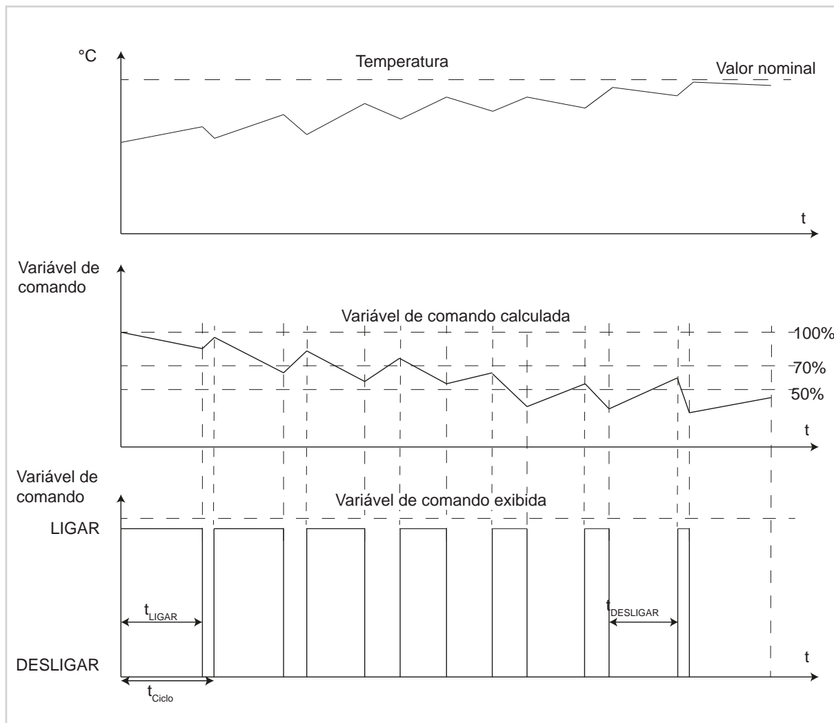
Figura 19: Regulação comutadora PI (MAP)
