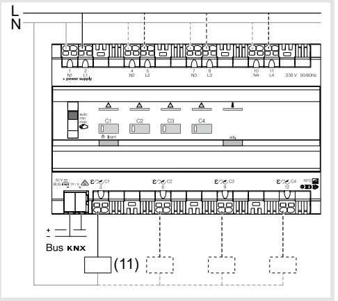
Afb. 3 : apparaat aansluiten eenfasig
