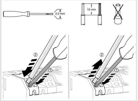
Afb. 2 : installatie/deinstallatie met steekklemmen
