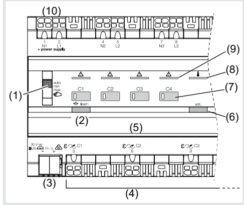
Afb. 1 : overzicht apparaten
