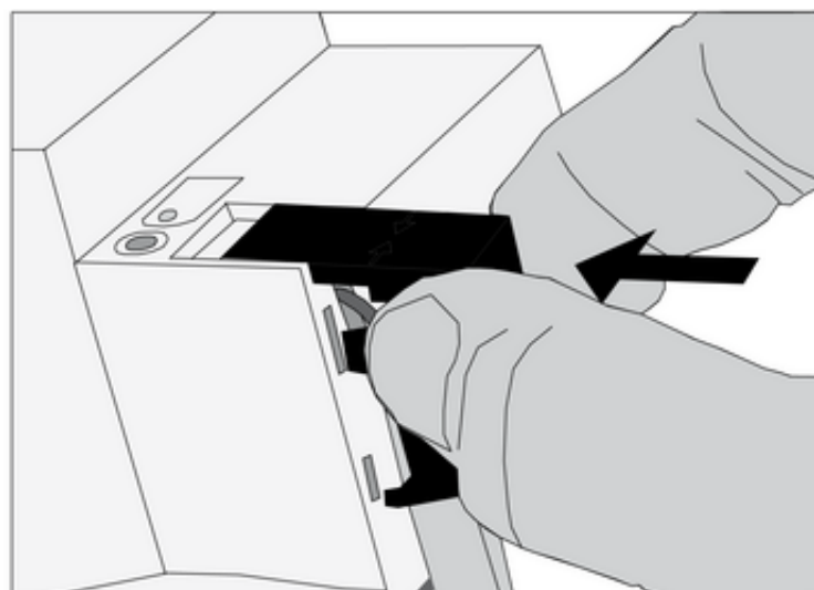
Bild 6: Abdeckkappe aufstecken
