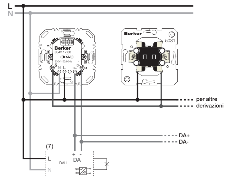
Figura 4: schema di collegamento con pulsante (contatto di chiusura) come derivazione
