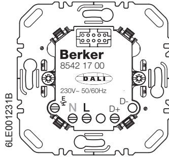
8542 17 00 DALI/DSI Steuereinsatz Inserto di comando DALI/DSI
