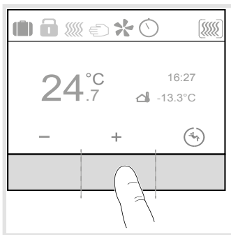
Figure 5 : Zones sensorielles de la surface de commande tactile
