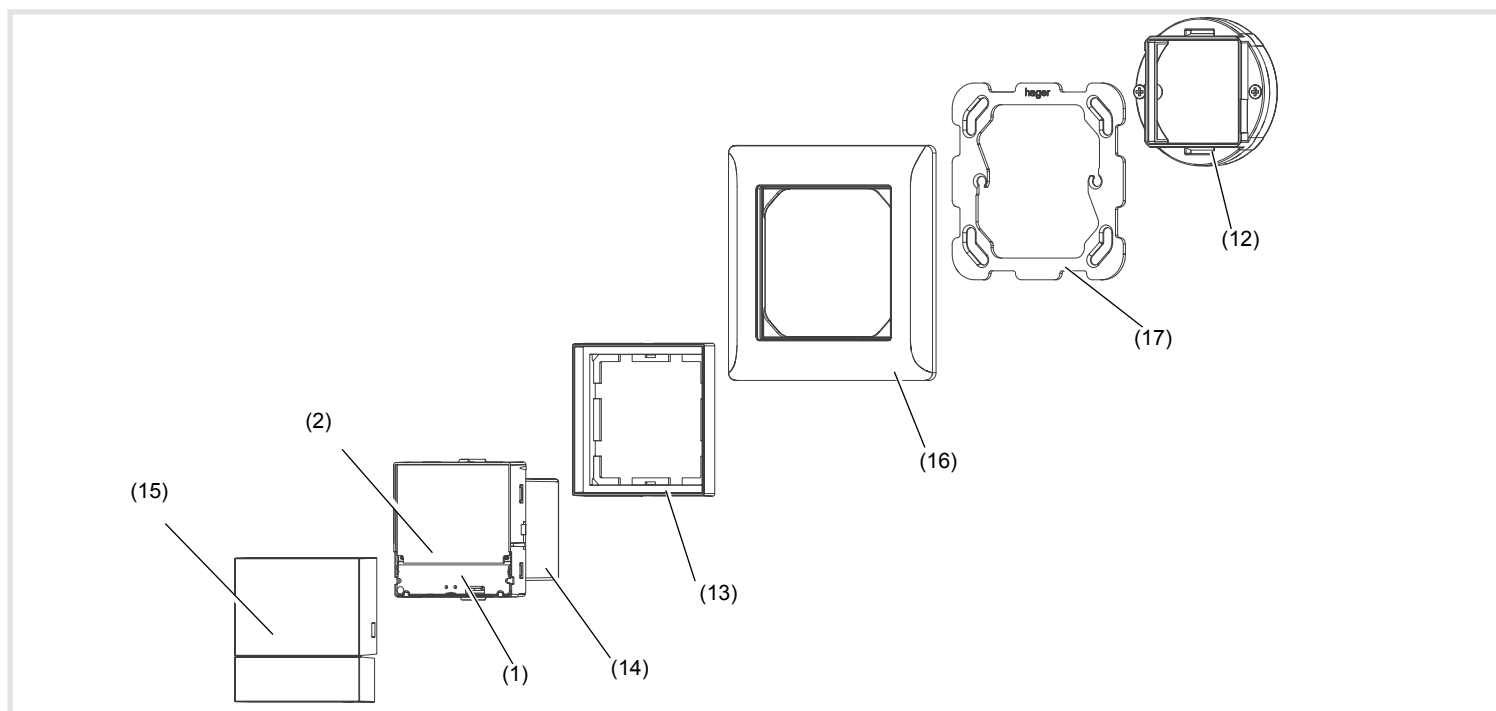
Image 19 : assemblage de l'appareil
