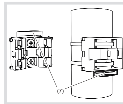
Bild 5: Wand- (links)/Mastbefestigung (rechts)
