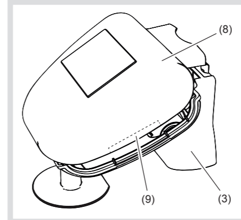
Bild 6: Montagevorbereitung
