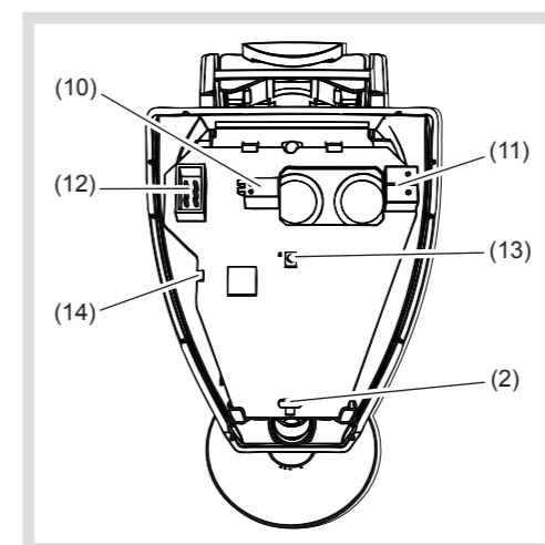
Figura 7: vista interna
