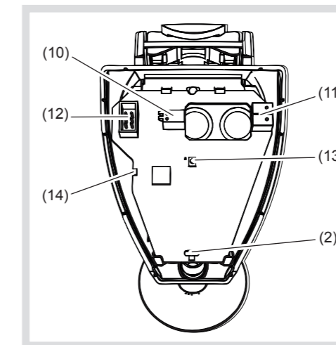
Bild 7: Innenansicht
