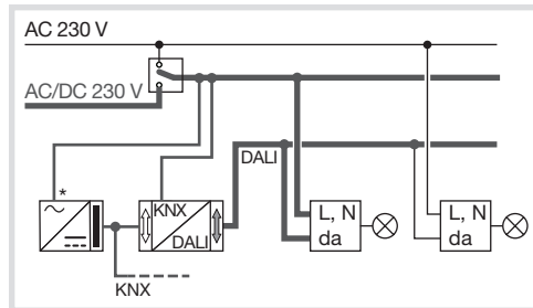
Figura 2: Iluminação de emergência, alimentação KNX e Gateway DALI alimentados pelo circuito central de alimentação de emergência
