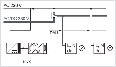
Figura 2: Alumbrado de emergencia, alimentación KNX y Pasarela DALI alimentada por el circuito central de alimentación de seguridad.
