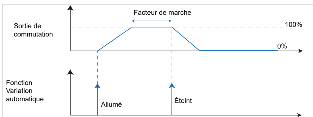
Image 28: Diagramme signal-temps Variation automatique
