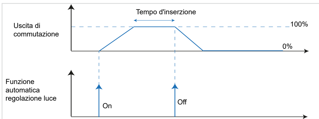
Figura 28: Diagramma segnale-tempo Funzione automatica regolazione luce
