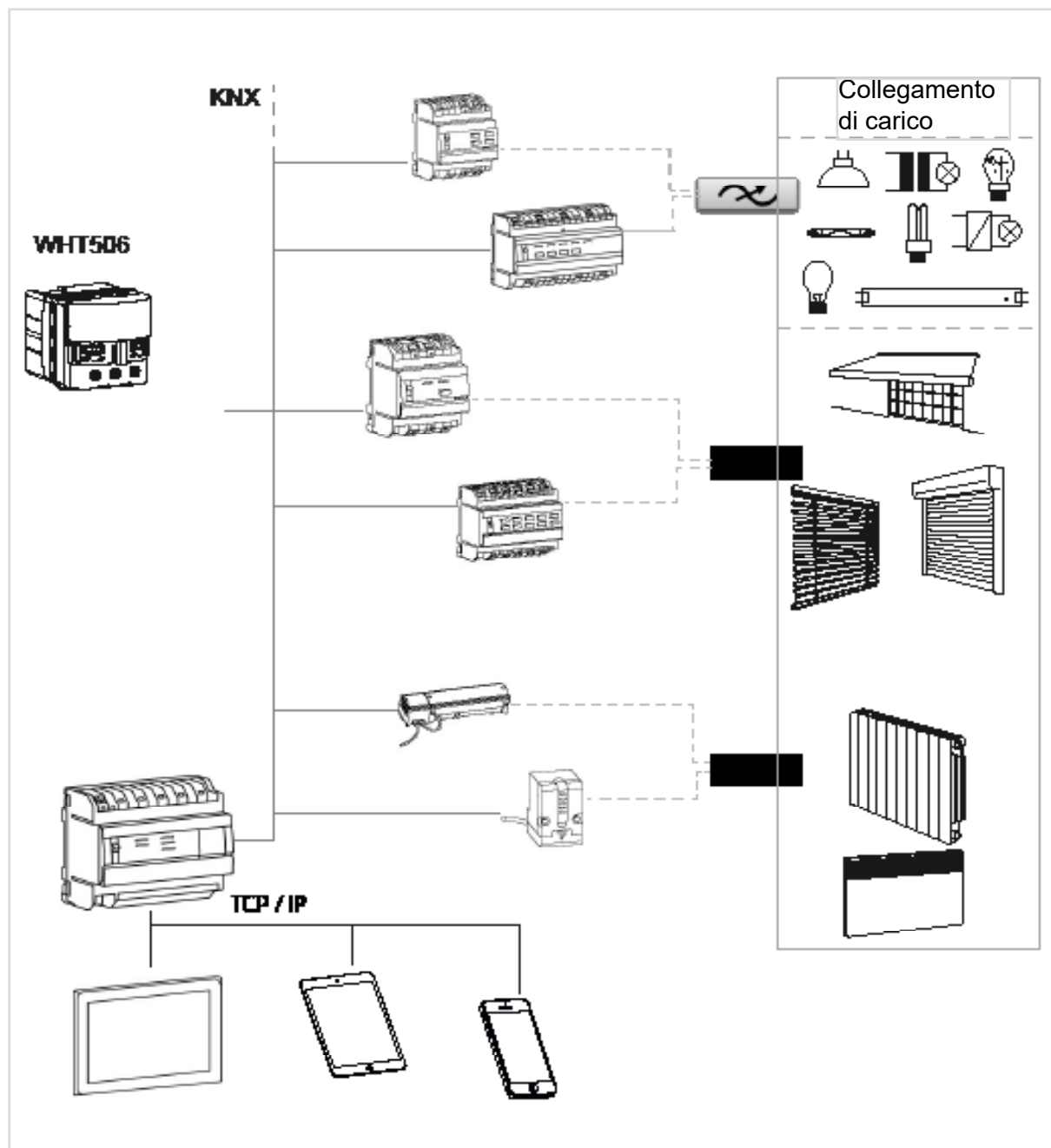
Figura 1: Panoramica dell'apparecchio
