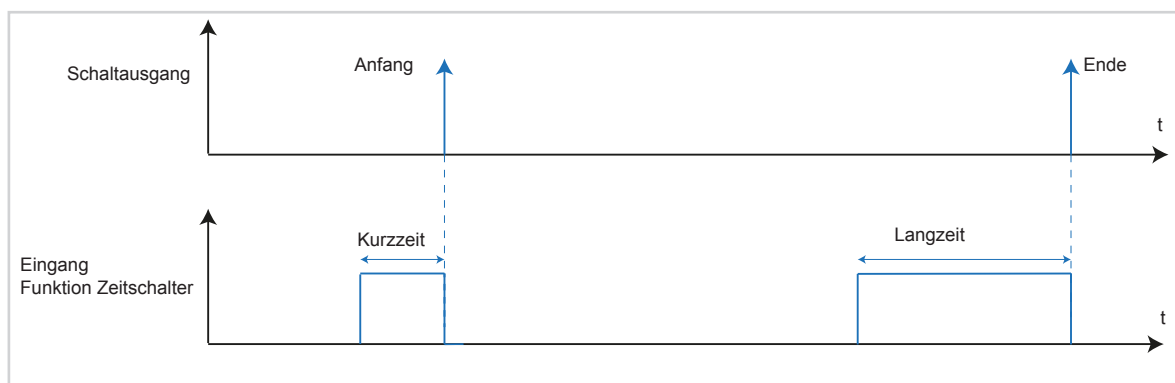
Bild 19: Signal-Zeit-Diagramm Zeitschalter
