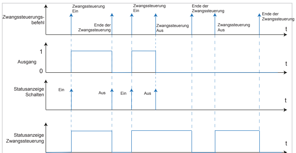
Bild 22: Signal-Zeit-Diagramm Zwangssteuerung
