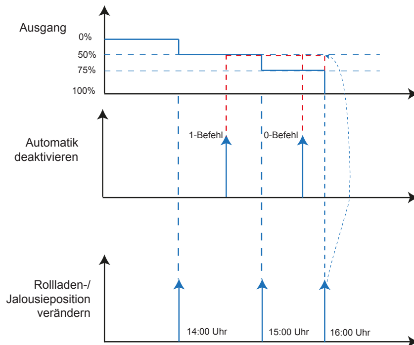
Bild 53: Signal-Zeit-Diagramm Automatik deaktivieren
