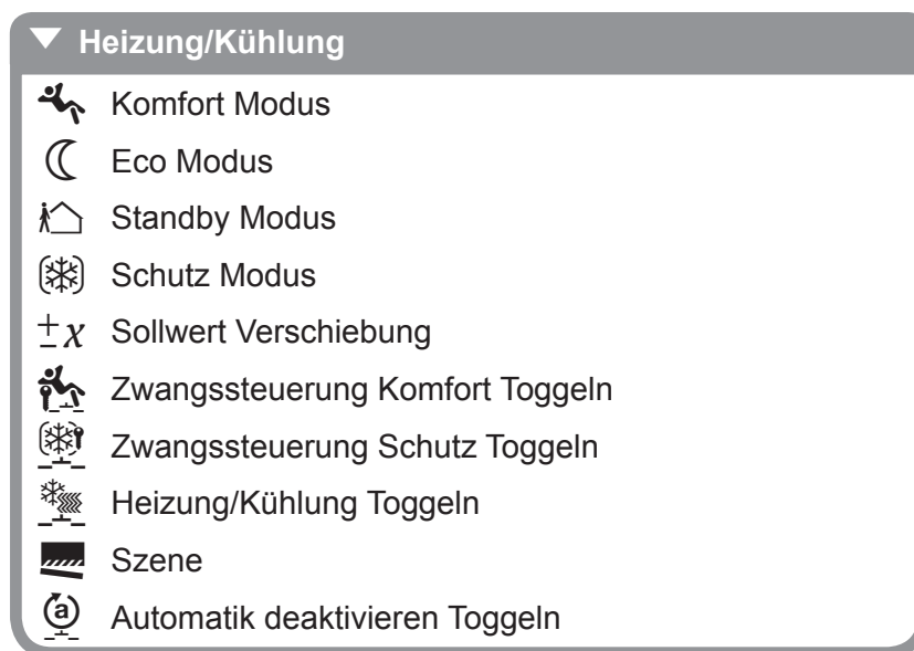
Bild 55: Funktionsübersicht Heizung/Kühlung
