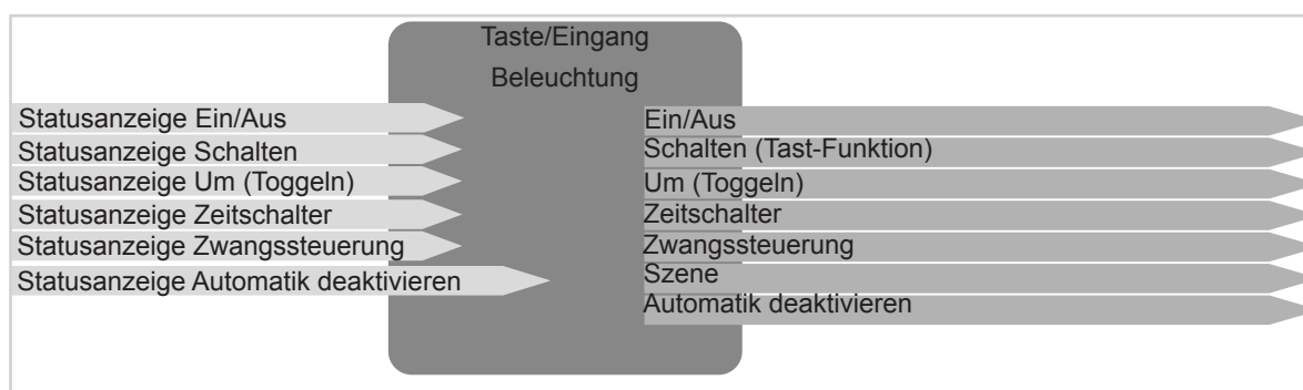
Bild 4: Ein-/Ausgangssignale Funktion Beleuchtung
