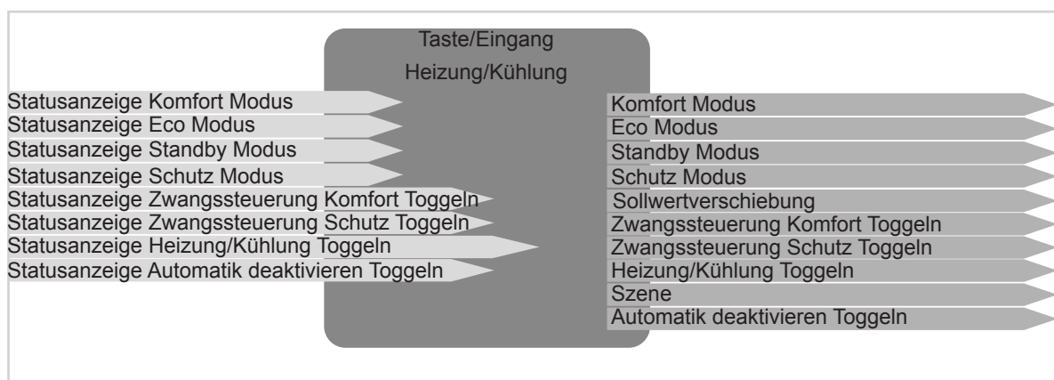
Bild 7: Ein-/Ausgangssignale Funktion Heizung/Kühlung
