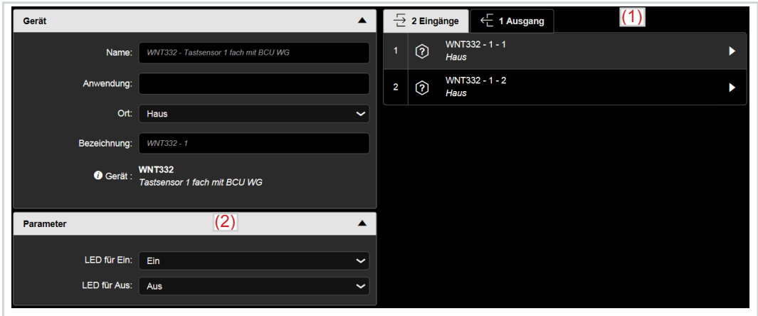
Bild 8: Geräteinformation
