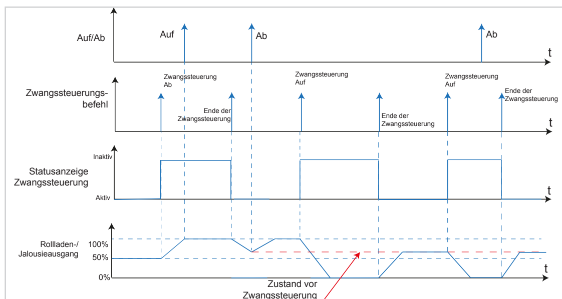
Bild 51: Signal-Zeit-Diagramm Zwangssteuerung Rolllade/Jalousie
