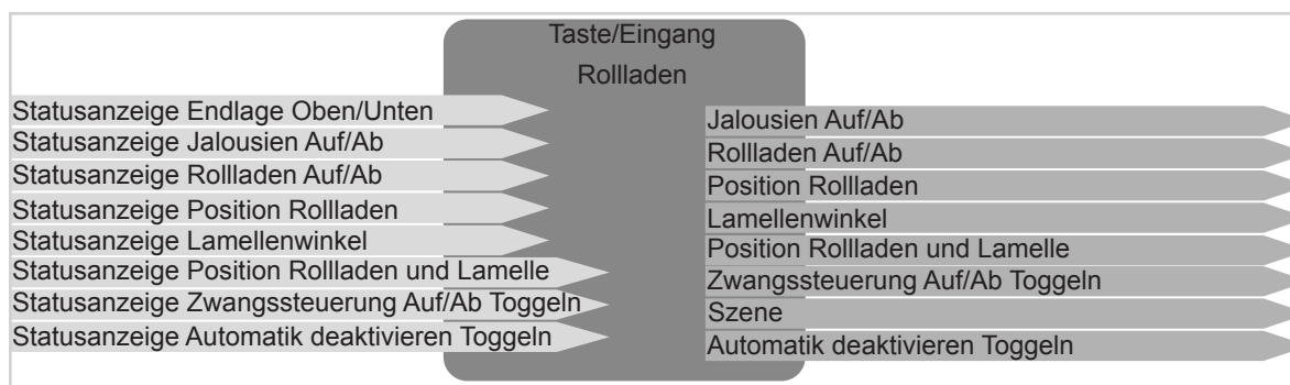
Bild 6: Ein-/Ausgangssignale Funktion Rollladen
