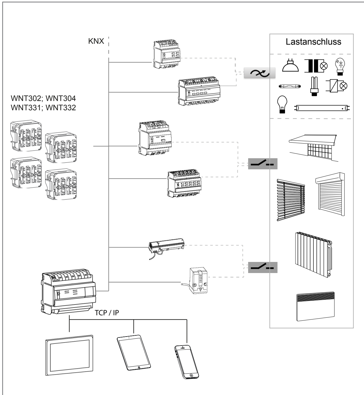
Bild 1: Geräteübersicht
