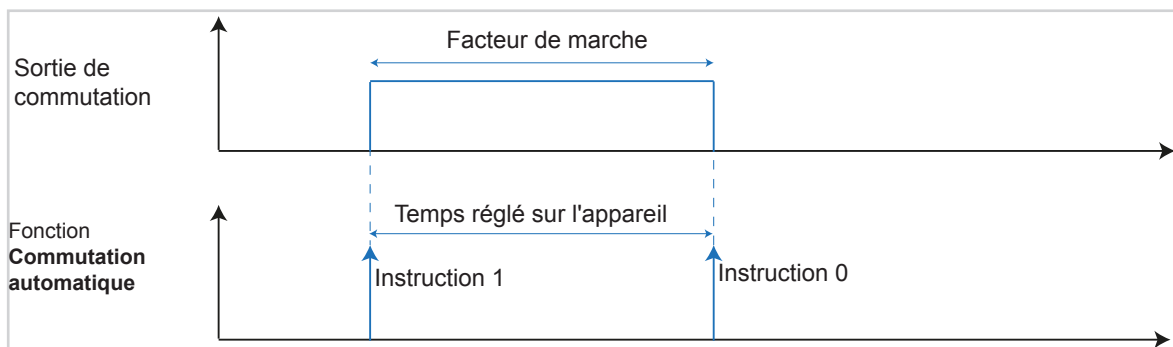
Image 17: Diagramme signal-temps Commutation automatique
