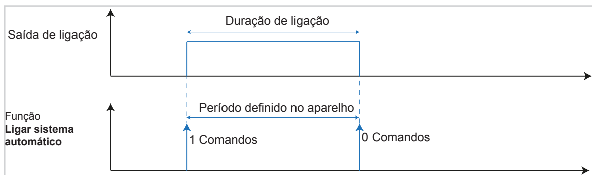
Figura 17: Diagrama de sinal e tempo Ligar sistema automático
