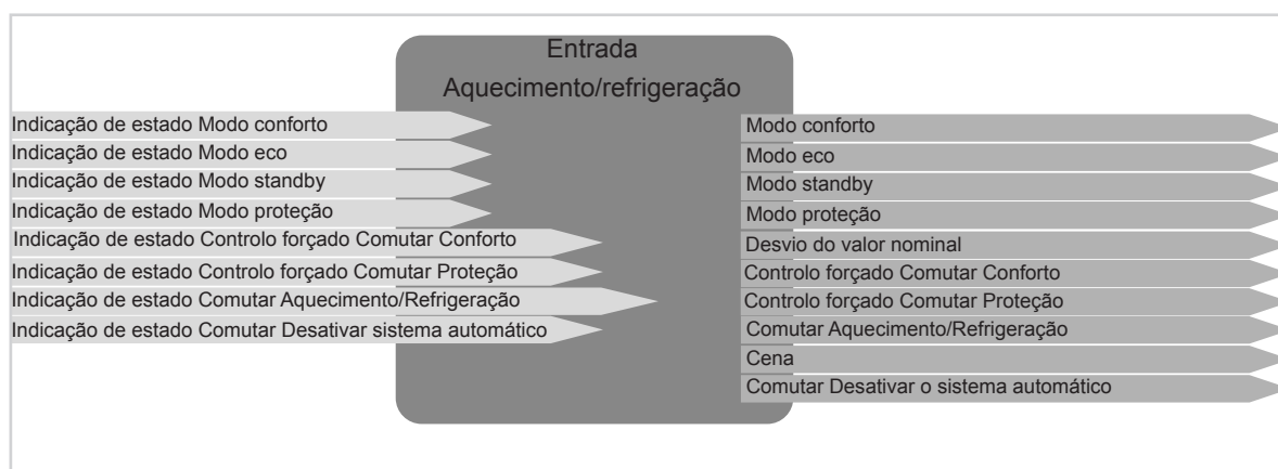
Figura 5: Sinais de entrada/saída Função aquecimento/refrigeração
