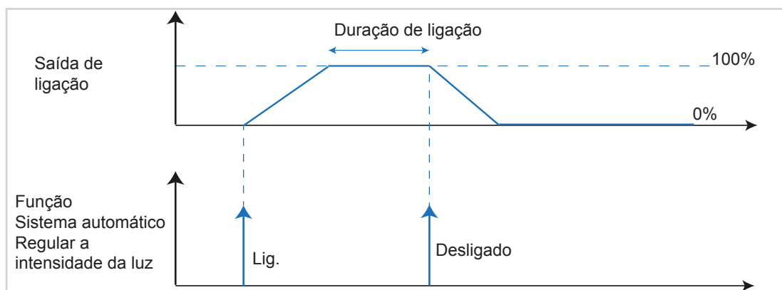
Figura 28: Diagrama de sinal e tempo Sistema automático Regular a intensidade da luz
