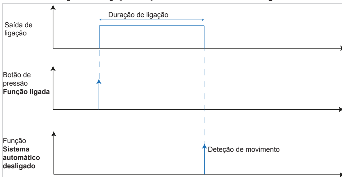
Figura 15: Diagrama de sinal e tempo Sistema automático desligado
