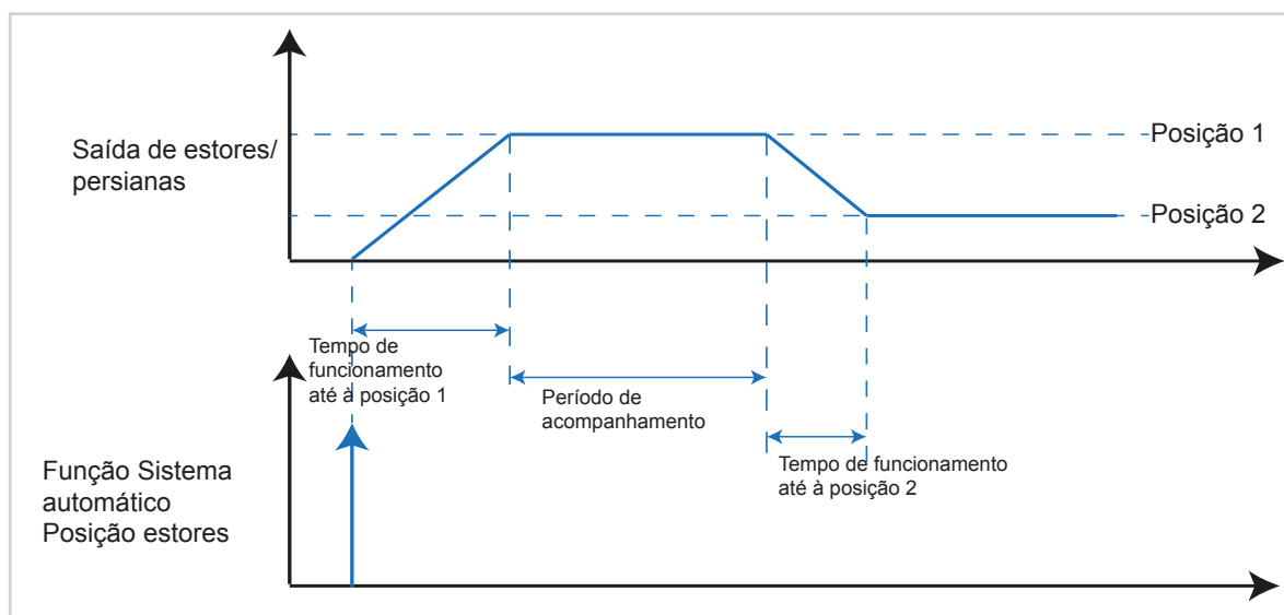
Figura 53: Diagrama de sinal e tempo Sistema automático Posição estores
