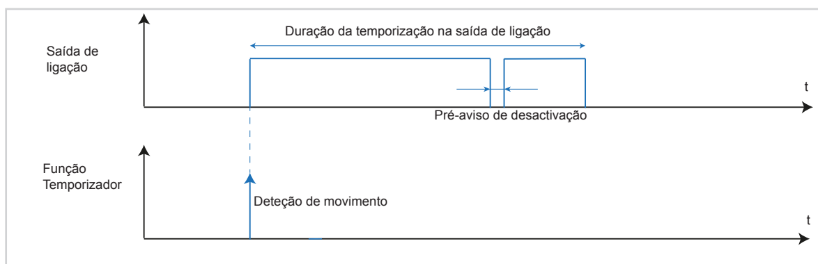
Figura 11: Diagrama de sinal e tempo Temporizador
