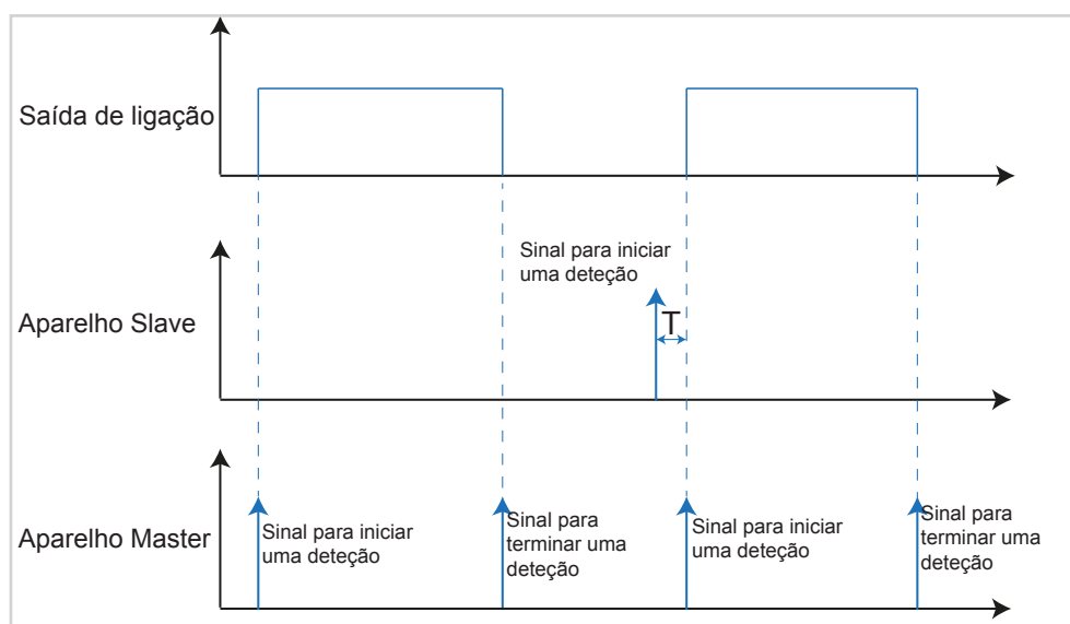
Figura 70: Diagrama de sinal e tempo Aplicação Master - Slave
