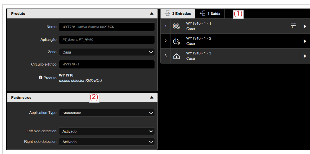
Figura 6: Informação relativa ao aparelho
