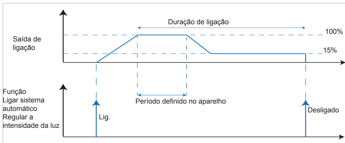
Figura 31: Diagrama de sinal e tempo Ligar sistema automático Regular a intensidade da luz
