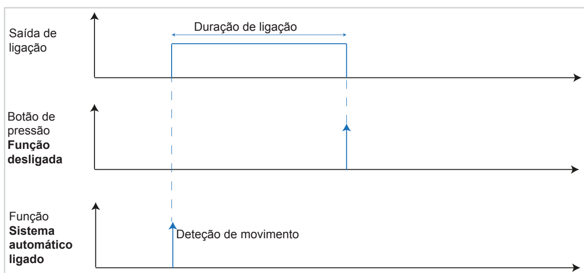
Figura 13: Diagrama de sinal e tempo Sistema automático ligado
