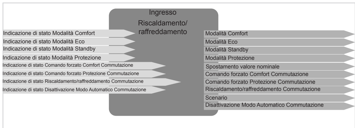
Figura 5: Segnali di ingresso/uscita funzione Riscaldamento/raffreddamento
