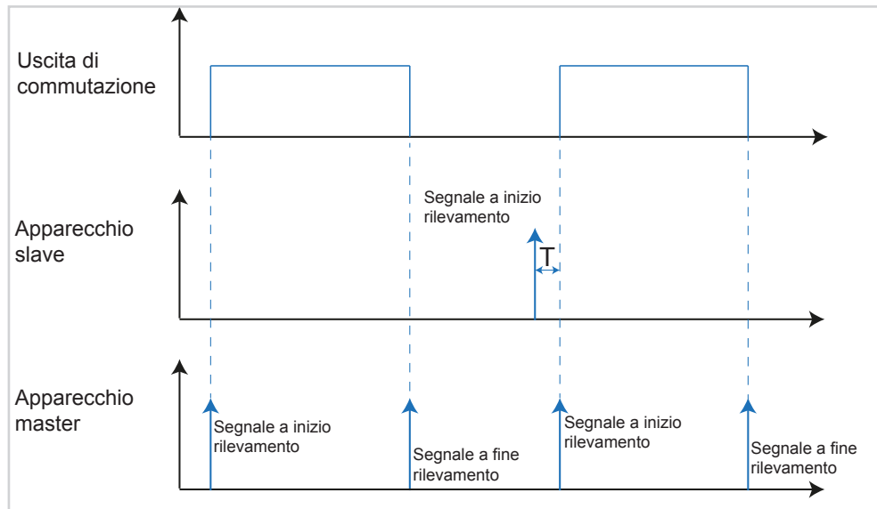
Figura 70: Diagramma segnale-tempo applicazione master - slave
