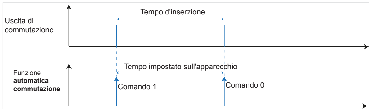
Figura 17: Diagramma segnale-tempo Funzione automatica commutazione
