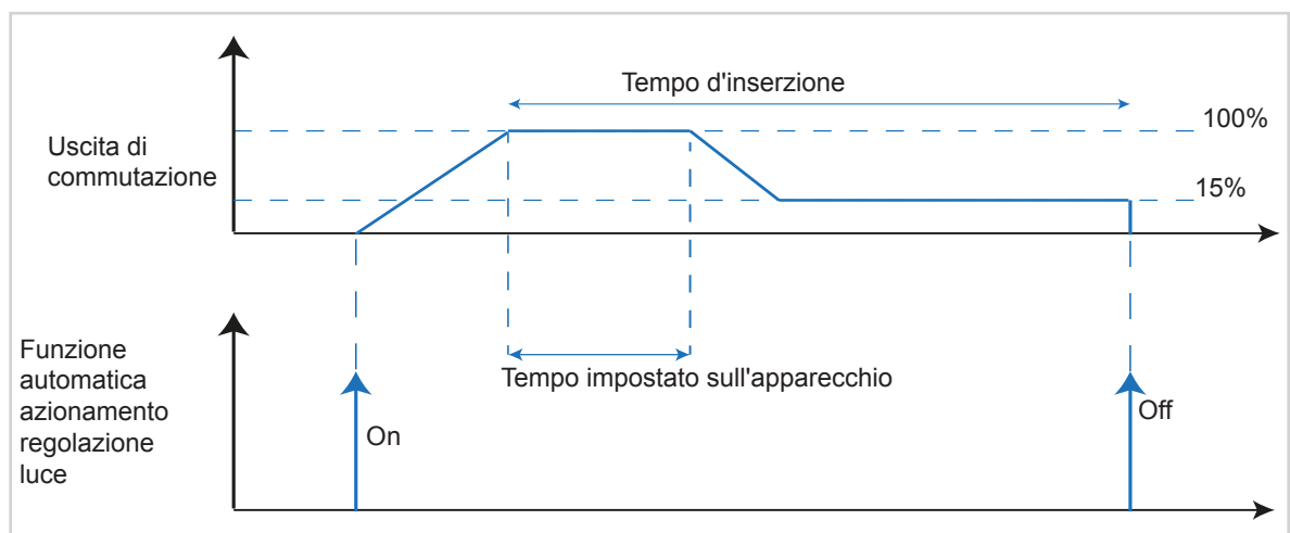
Figura 31: Diagramma segnale-tempo Funzione automatica azionamento regolazione luce
