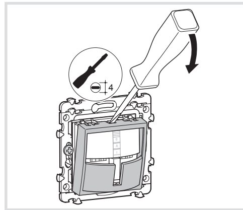
Afb. 8: demontage van de afdekking
