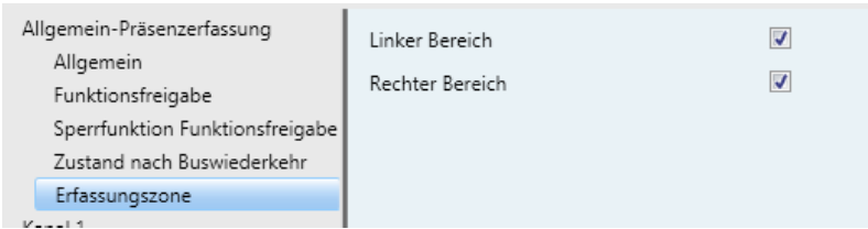
Bild 6: Allgemein „Erfassungszone“
