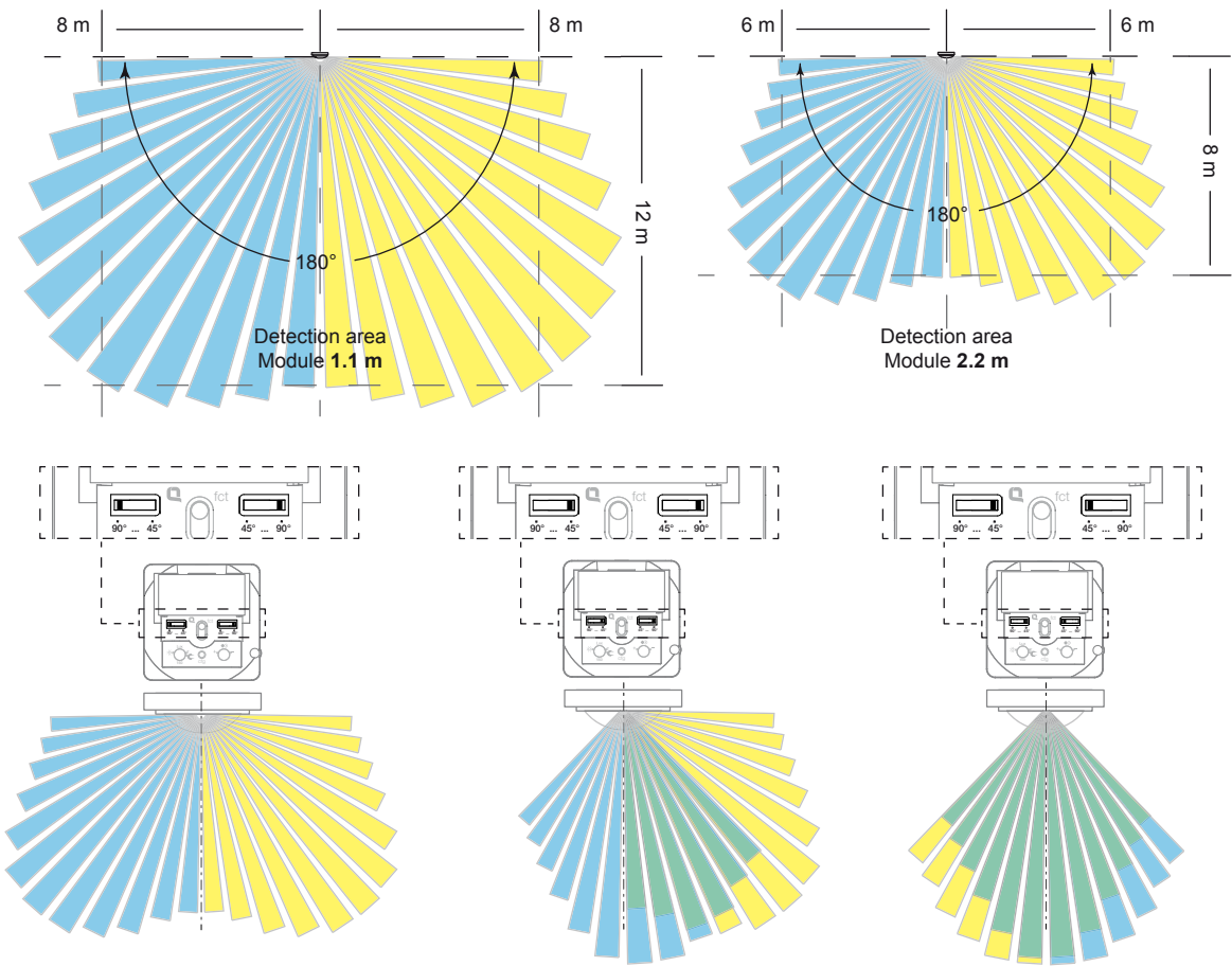
Bild 7: Erfassungsbereiche
