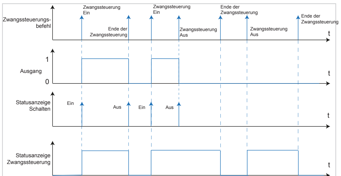
Bild 24: Signal-Zeit-Diagramm Zwangssteuerung
