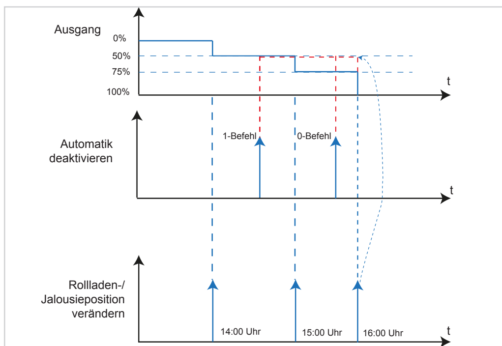
Bild 55: Signal-Zeit-Diagramm Automatik deaktivieren
