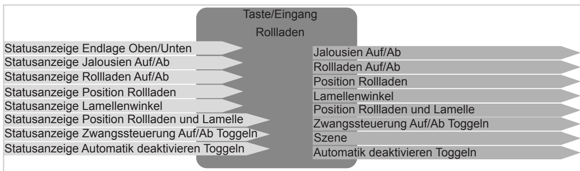
Bild 5: Ein-/Ausgangssignale Funktion Rollläden
