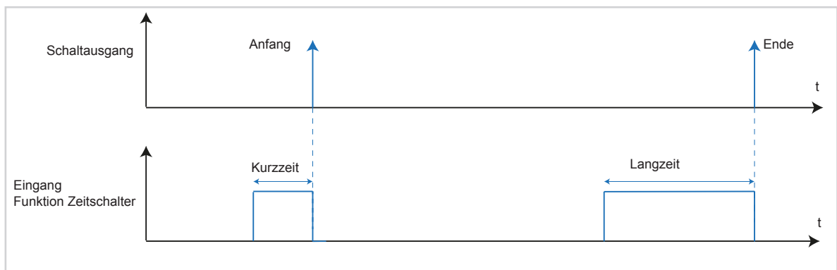
Bild 21: Signal-Zeit-Diagramm Zeitschalter
