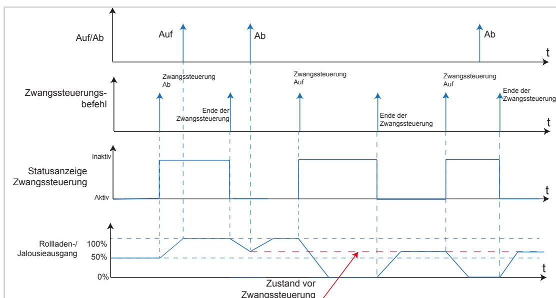
Bild 53: Signal-Zeit-Diagramm Zwangssteuerung Rolllade/Jalousie
