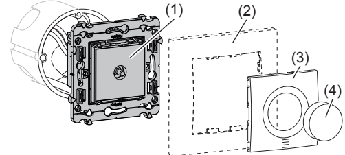
Bild 2: Tastdimmer WK061
