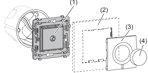
Bild 1: Drehdimmer WK060
