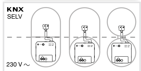
Figura 2: installazione con punto di collegamento separato
