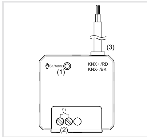
Figura 1: vista dell'apparecchio
