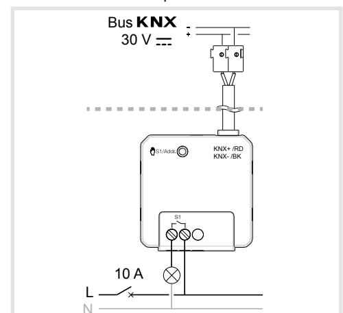
Figura 3: collegamento dell'apparecchio singolo Rispettare le direttive di installazione per la tensione SELV. Mantenere una distanza minima di 4 mm tra la tensione di rete e i fili del bus.
