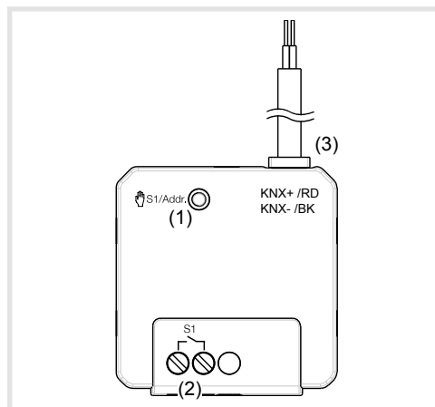
Bild 1: Geräteübersicht
