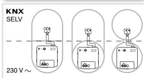
Bild 2: Installation mit getrenntem Anschlussraum
