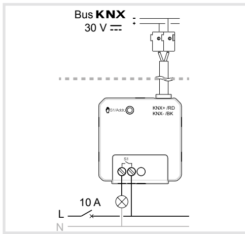
Bild 3: Geräteanschluss 1fach
