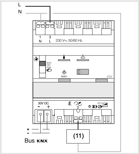
Figura 3: Collegamento dell'apparecchio
