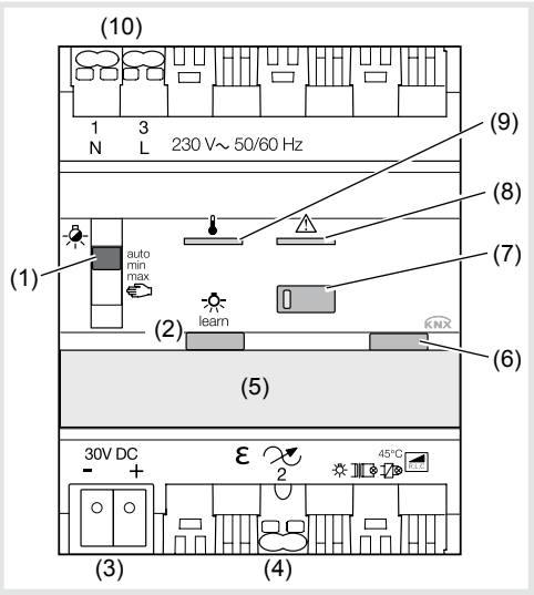
Figura 1: Vista dell'apparecchio
