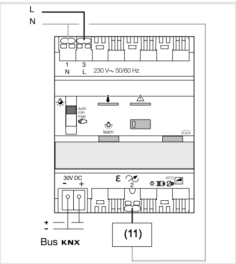
Bild 3: Geräteanschluss
