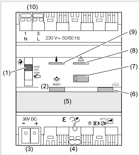
Bild 1: Geräteübersicht
