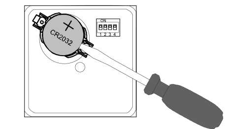
Afbeelding 4: Batterij verwijderen
