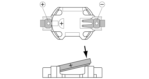
Bild 5: Batterie einlegen
