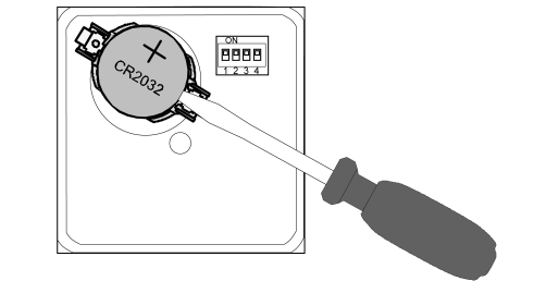
Bild 4: Batterie entfernen
