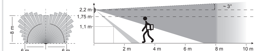
Bild 7: Erfassungsbereich des Bewegungsmelders Montagehöhe 2,2 m
