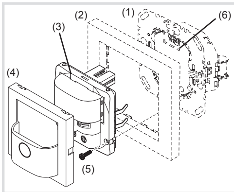
Bild 1: Geräteaufbau
