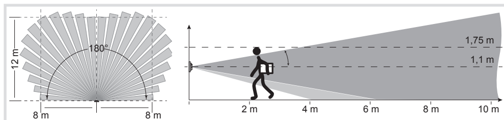
Bild 6: Erfassungsbereich des Bewegungsmelders Montagehöhe 1,1 m
