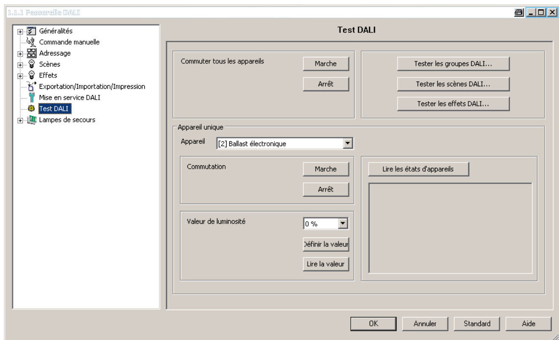
Figure 73: Environnement de test DALI dans le plug-in ETS3
