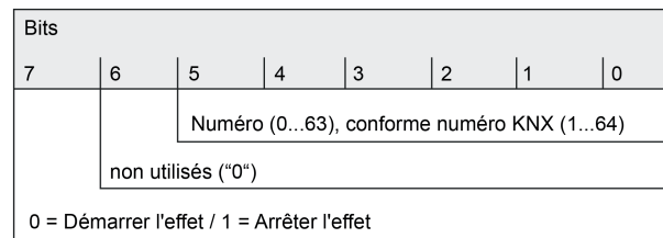
Figure 54: Structure de la valeur d'objet pour le poste auxiliaire d'effet
