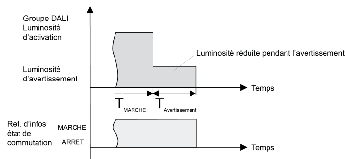
Figure 43: La fonction d'avertissement de la fonction cage d'escalier sans fonction ARRÊT progressif
