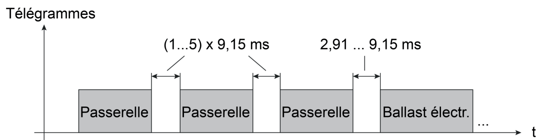
Figure 28: Temps de pause entre les télégrammes DALI
