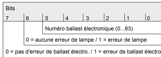
Figure 29: Structure du télégramme État d'erreur 1 octet
