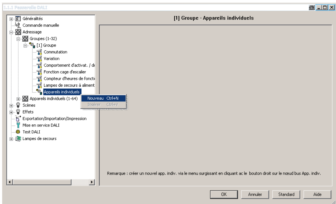
Figure 70: Affectation d'un ballast électronique à un groupe - Mise en service hors ligne
