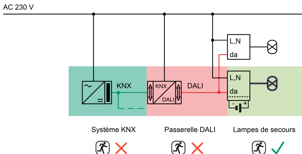
Figure 20: Exemple d'application avec lampes de secours DALI autonomes
