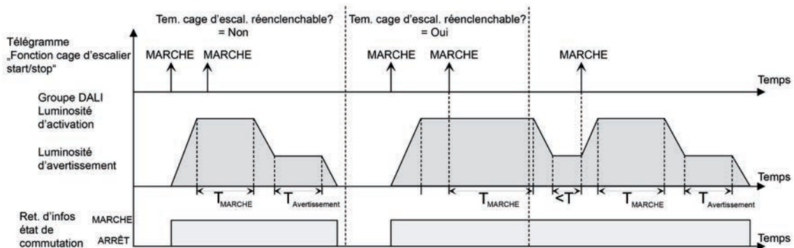
Figure 44: Comportement d'activation de la fonction cage d'escalier avec fonctions progressives (exemple avec luminosité minimale = 0 %)
