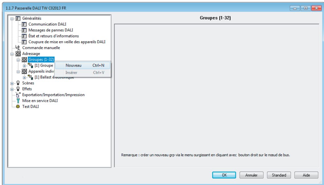
Figure 20: Ajout de groupes DALI (identique pour les appareils individuels)
