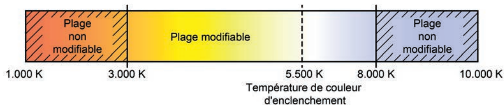
Figure 35: Exemple d'une plage de température de couleur configurée avec une température de couleur d'enclenchement
