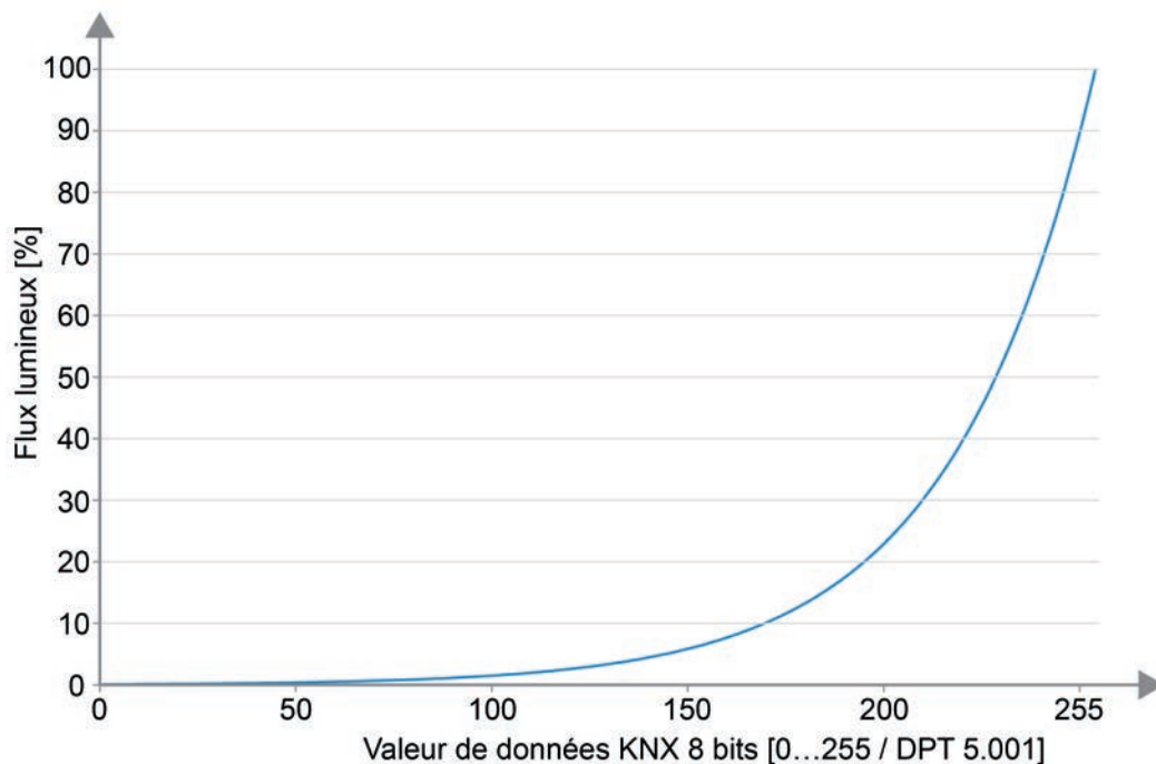
Figure 34: Courbe caractéristique de variation DALI logarithmique (flux lumineux relatif [%] en fonction de la valeur de données KNX de 8 bits [0...255])
