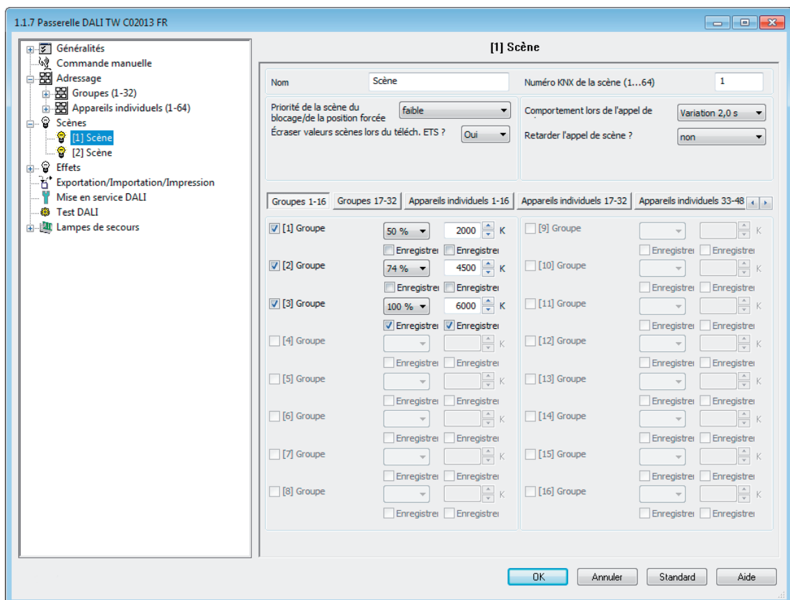
Figure 53: Page de configuration d'une scène à titre d'exemple avec deux scènes créées et trois groupes DALI
