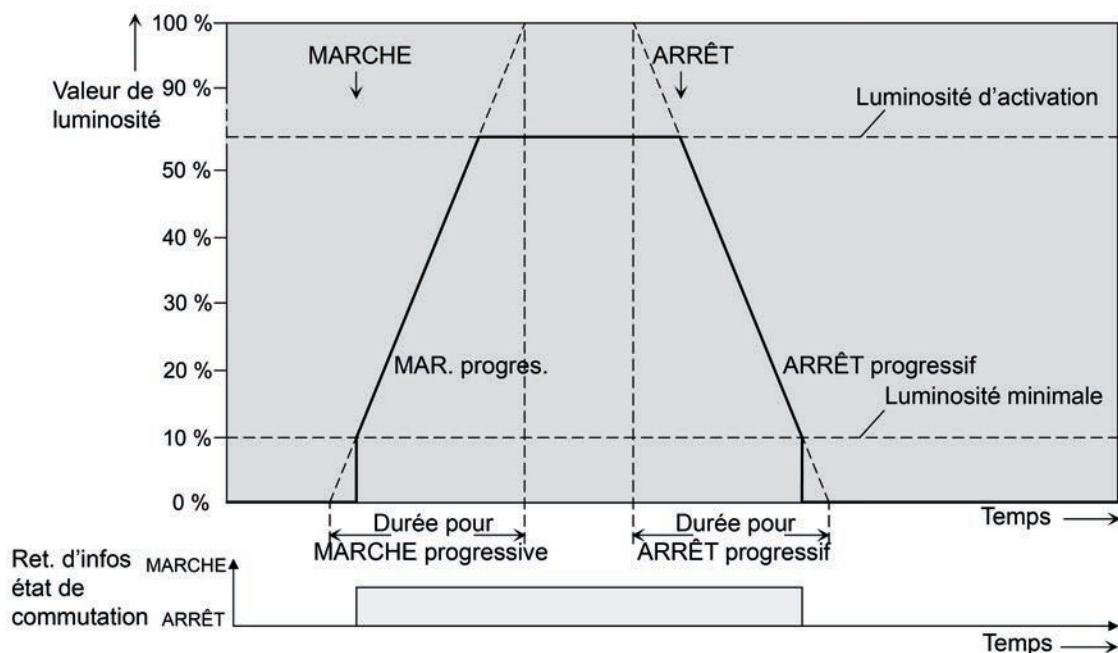
Figure 42: Exemple de comportement de variation des fonctions MARCHÉ progressive / ARRÊT progressif avec luminosité minimale > 0 %
