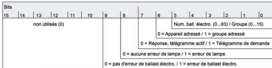
Figure 27: Structure du télégramme État d'erreur KNX 2 octets
