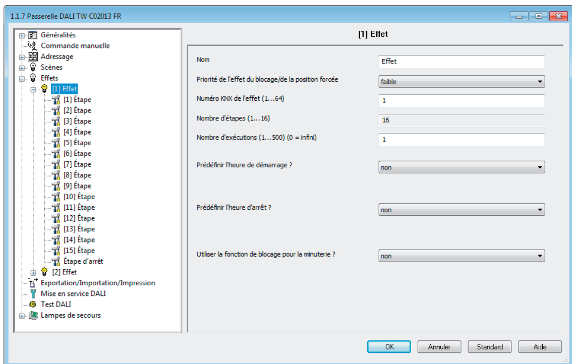
Figure 55: Exemple de page de configuration d'un effet avec 15 étapes d'effet créées et l'étape d'arrêt
