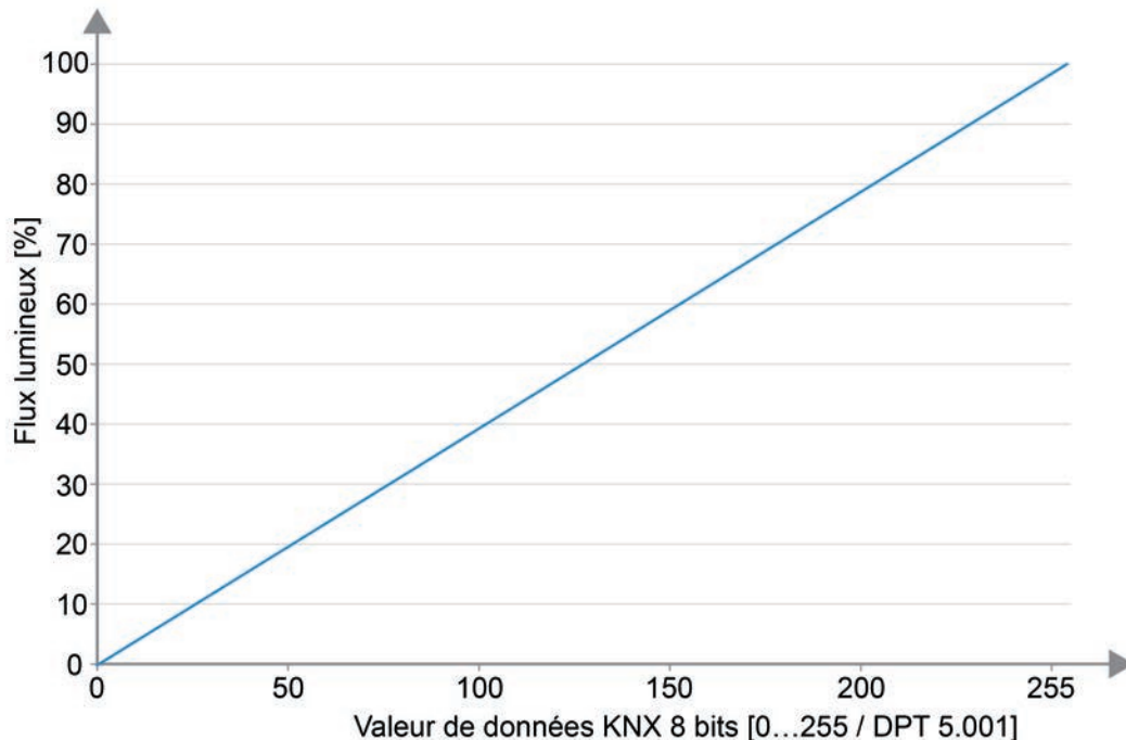
Figure 33: Courbe caractéristique de variation DALI linéaire (flux lumineux relatif [%] en fonction de la valeur de données KNX de 8 bits [0...255])
