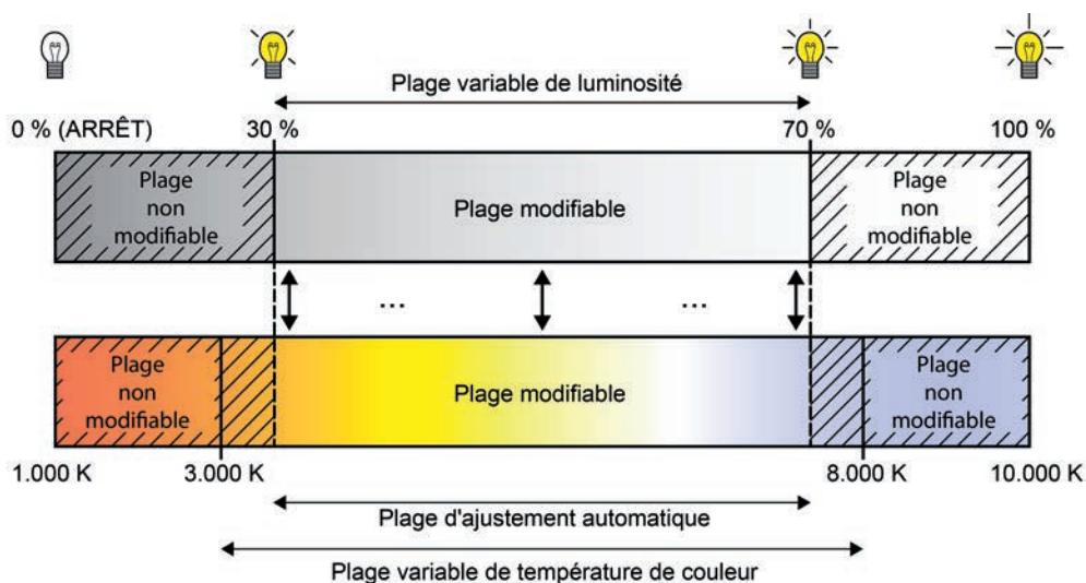
Figure 38: Adaptation automatique de la température de couleur à la luminosité réglée Exemple avec une plage de luminosité et de température de couleur restreinte
