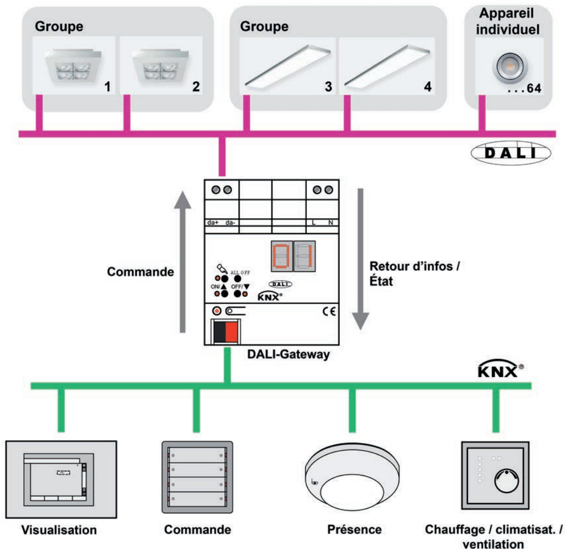
Figure 9: Aperçu du principe de connexion d'un système DALI KNX (exemple)
