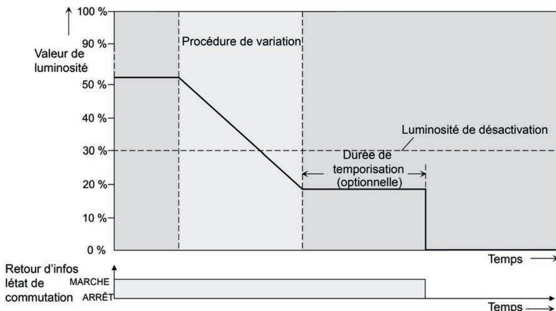
Figure 41: Comportement de variation et de commutation de la fonction de désactivation automatique
