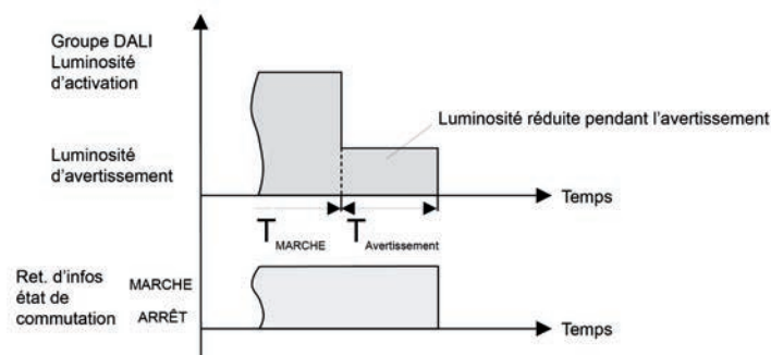
Figure 47: La fonction d'avertissement de la fonction cage d'escalier sans fonction ARRÊT progressif
