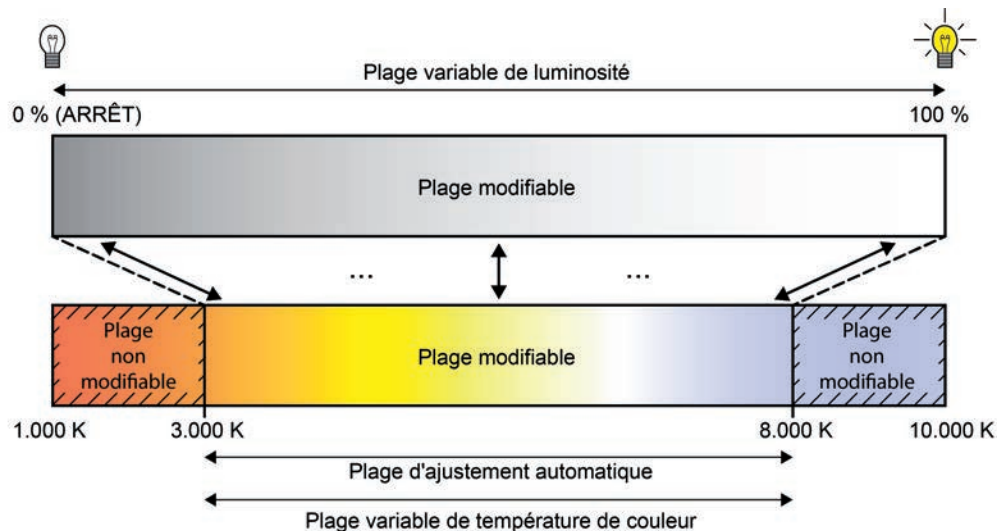
Figure 39: Adaptation automatique de la température de couleur à la luminosité réglée Exemple avec une plage de température de couleur restreinte
