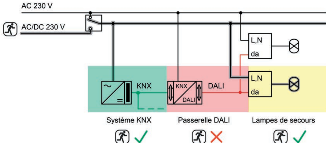
Figure 17: Exemple d'alimentation centralisée - Équipements DALI et système KNX intégrés dans l'alimentation de secours
