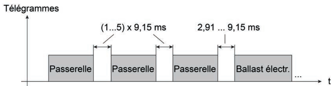
Figure 25: Temps de pause entre les télégrammes DALI
