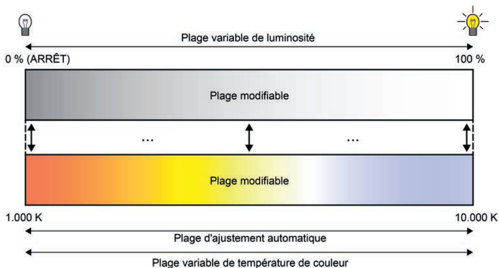
Figure 37: Adaptation automatique de la température de couleur à la luminosité réglée Exemple dans la plage de luminosité et de température de couleur maximale
