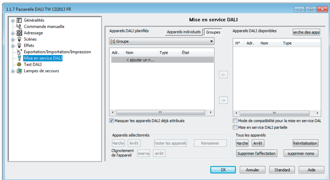
Figure 61: Environnement de mise en service DALI dans le plug-in ETS
