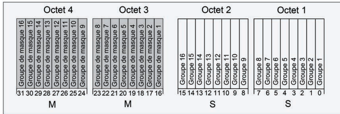
Figure 28: Structure des objets du retour d'infos global sur l'exemple de l'objet pour les groupes 1-16
