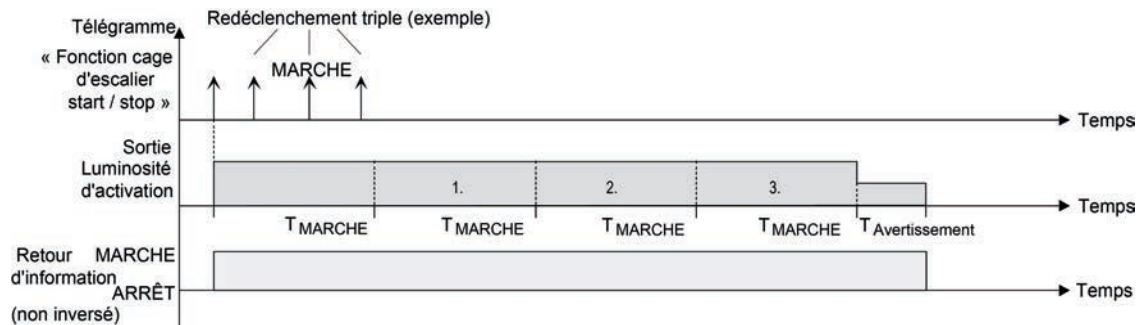
Figure 51: Prolongation de la fonction cage d'escalier
