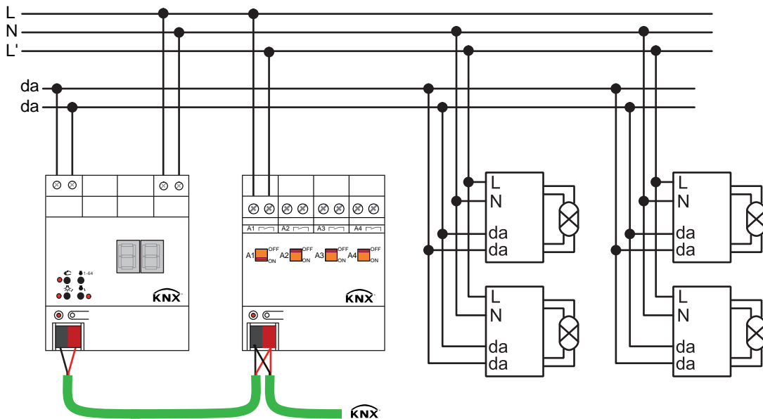
Figure 29: Exemple de schéma de raccordement pour la coupure de mise en service par un actionneur de commutation KNX
