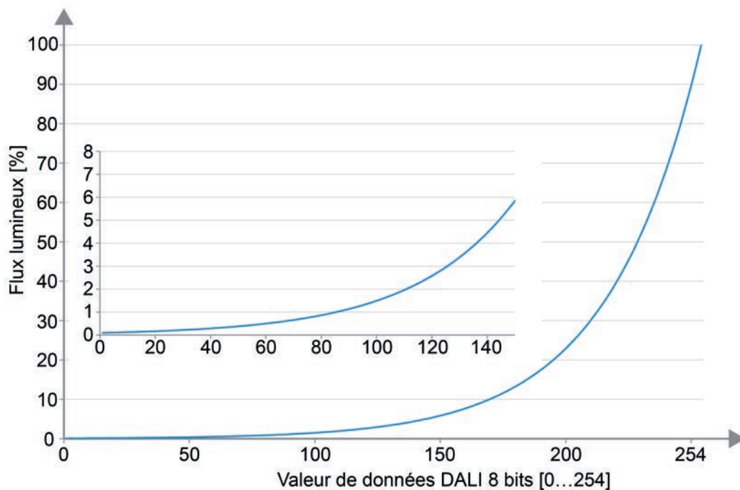
Figure 32: Courbe de variation logarithmique dans des équipements DALI (flux lumineux relatif [%] en fonction de la valeur de données DALI de 8 bits [0...254])
