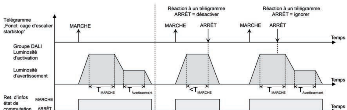
Figure 46: Comportement de désactivation de la fonction cage d'escalier avec fonctions progressives (exemple avec luminosité minimale = 0 %)
