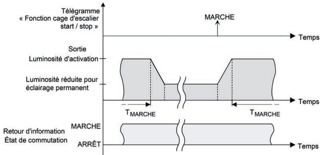
Figure 50: Éclairage permanent de la fonction cage d'escalier avec fonction ARRÊT progressif
