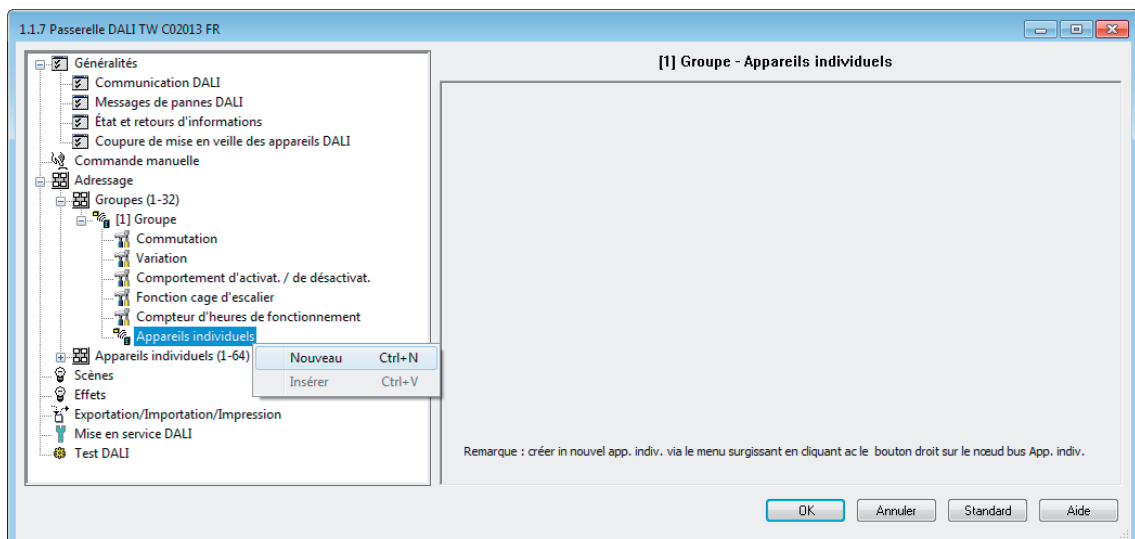
Figure 75: Affectation d'un ballast électronique à un groupe - Mise en service hors ligne
