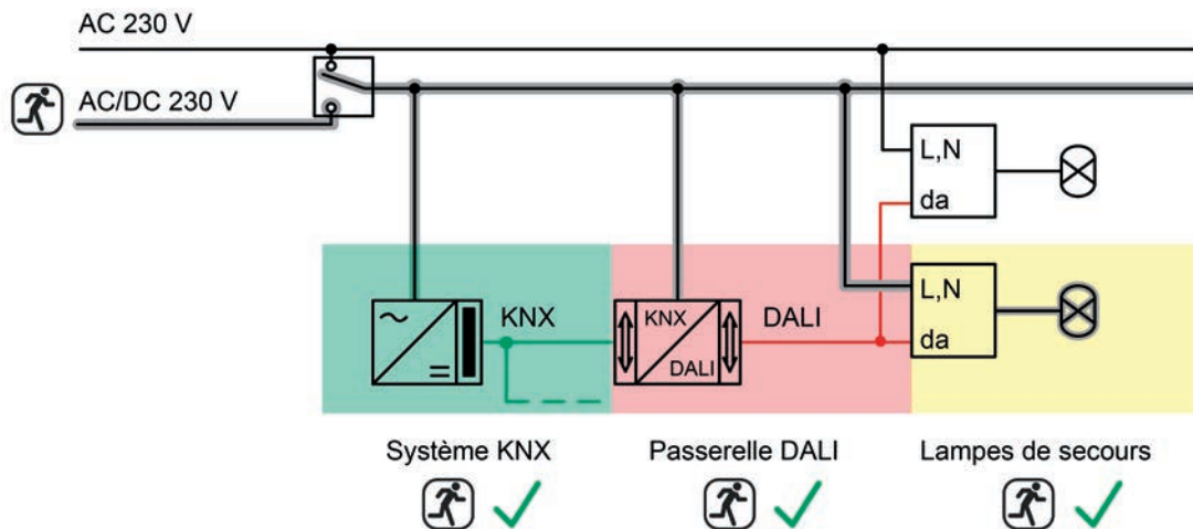
Figure 18: Exemple d'alimentation centralisée - Équipements DALI, système KNX et passerelle DALI intégrés dans l'alimentation de secours
