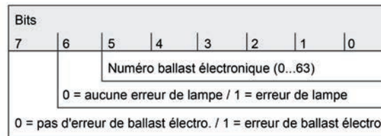
Figure 26: Structure du télégramme État d'erreur 1 octet
