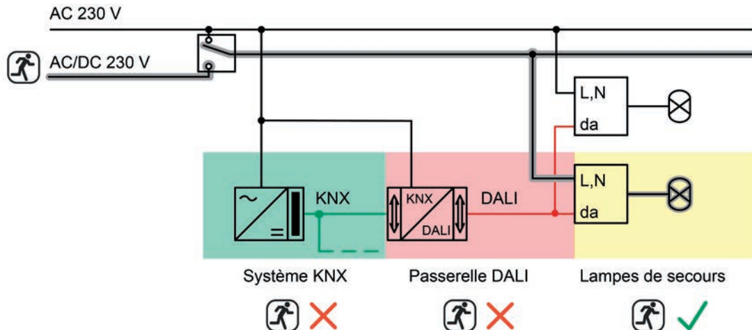
Figure 16: Exemple d'alimentation centralisée - Uniquement équipements DALI intégrés dans l'alimentation de secours
