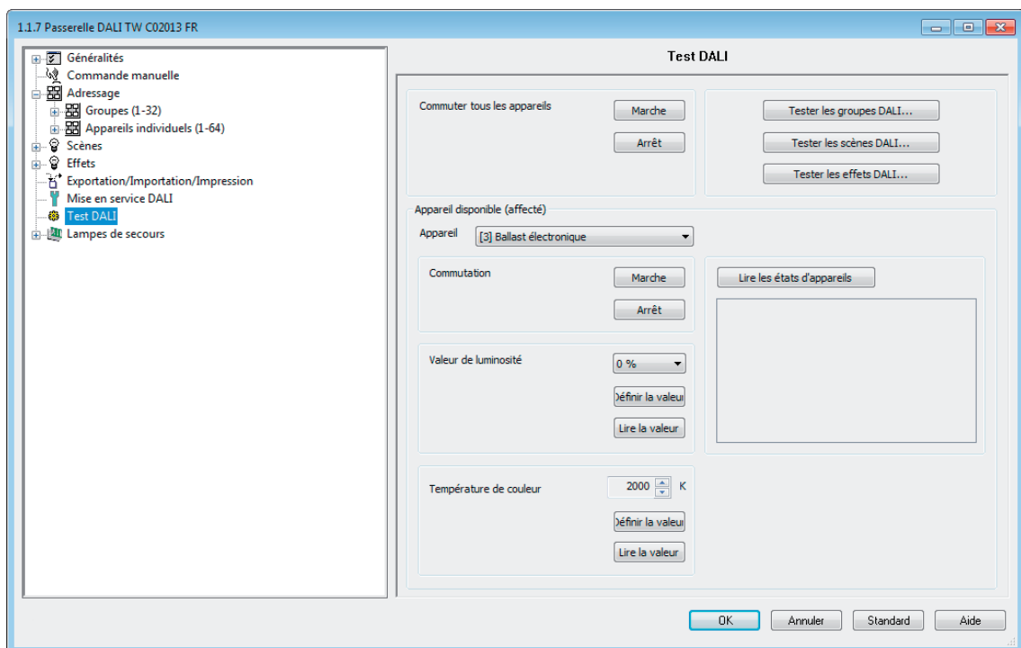
Figure 79: Environnement de test DALI dans le plug-in ETS
