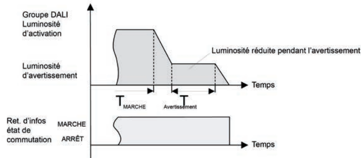
Figure 48: La fonction d'avertissement de la fonction cage d'escalier avec fonction ARRÊT progressif (exemple avec luminosité minimale = 0 %)
