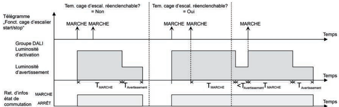
Figure 43: Comportement d'activation de la fonction cage d'escalier sans fonctions progressives
