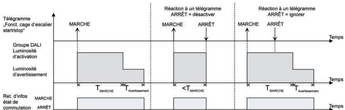
Figure 45: Comportement de désactivation de la fonction cage d'escalier sans fonctions progressives
