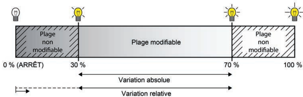
Figure 31: Exemple d'une plage de luminosité à intensité variable
