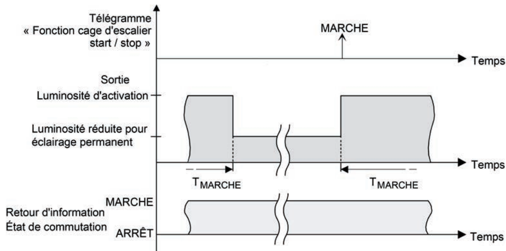
Figure 49: Éclairage permanent de la fonction cage d'escalier sans fonctions progressives
