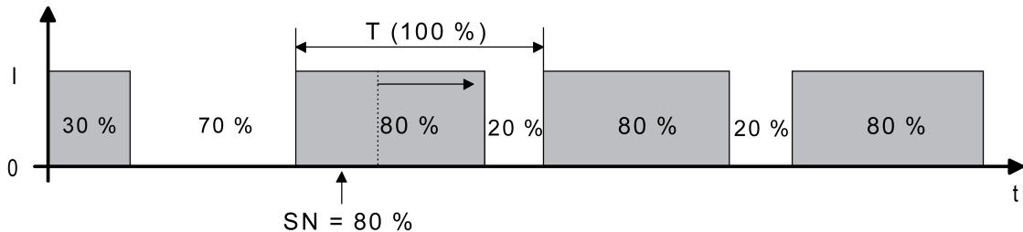
Bild 46: Stellgrößenänderung z. B. von 30 % auf 80 % während Öffnungsphase des Ventils
