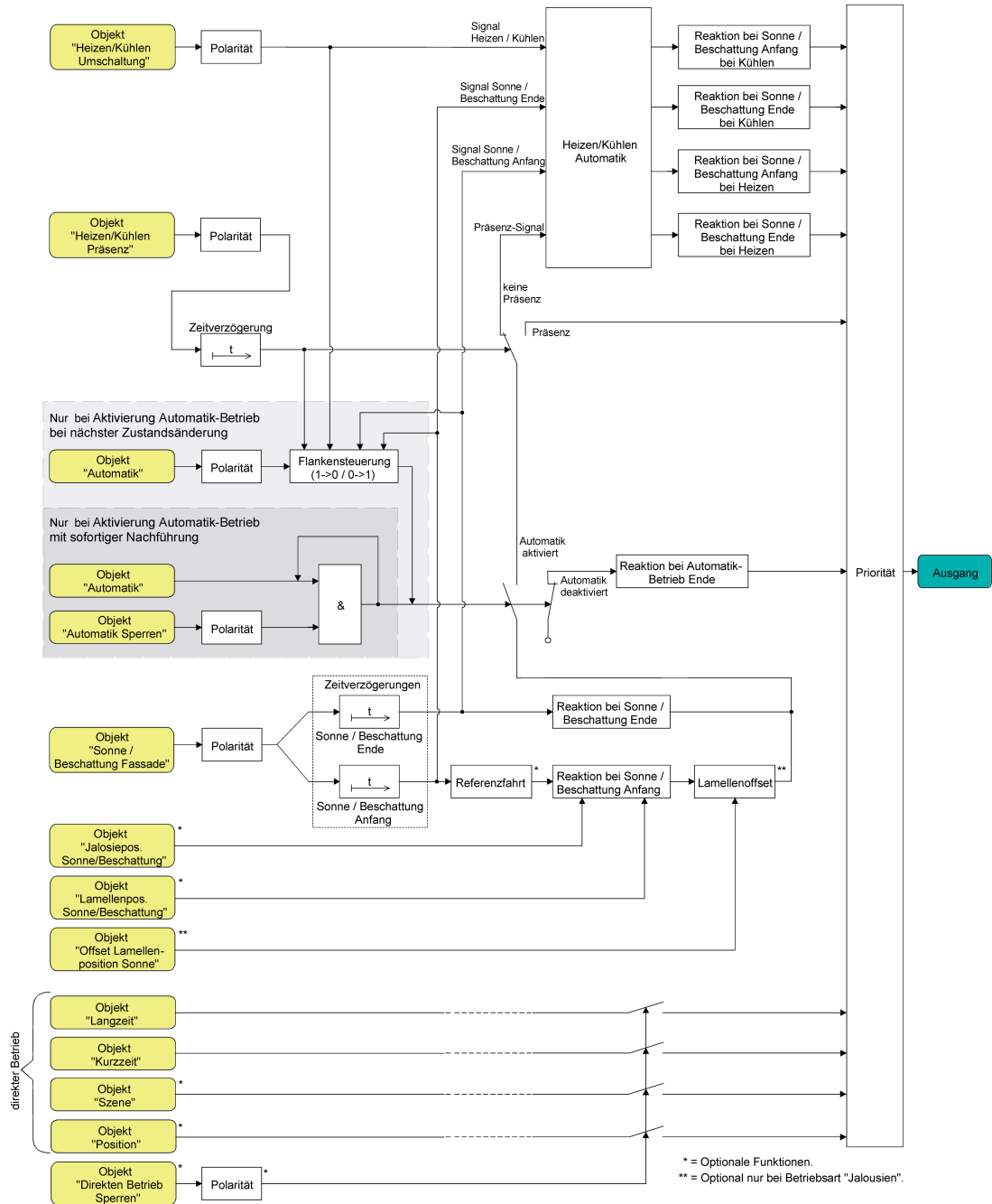
Bild 34: Funktionsschaltbild der Heizen/Kühlen-Automatik
