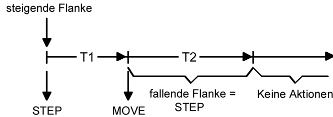
Bild 10: Bedienkonzept "Kurz-Lang-Kurz"
