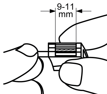
Bild 6: Abisolierlänge
