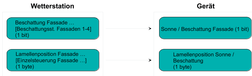
Bild 30: Projektierung der Kommunikationsobjekte für Anwendungsbeispiel III.
