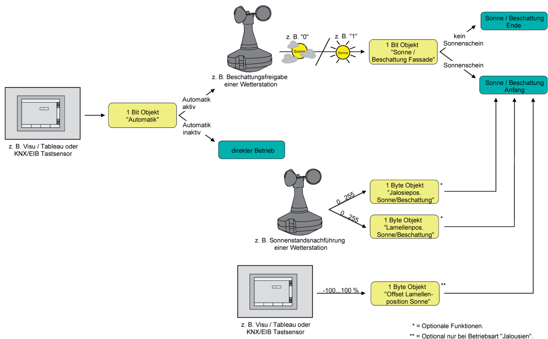
Bild 25: Prinzipschaltbild des erweiterten Sonnenschutzes (zur Vereinfachung ohne Sperrfunktionen)
