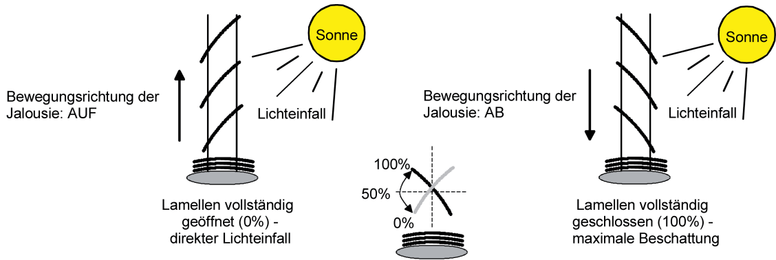
Bild 15: Typ 1 - Lamellenjalousien mit schräger Lamellenstellung in beide Fahrrichtungen
