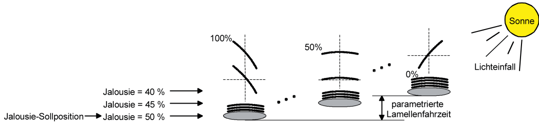
Bild 18: Beispiel für Lamellenpositionierung mit Auswirkung auf die Jalousieposition (Beispielhaft für Lamellentyp 1. Typ 2 sinngemäß gleich.)
