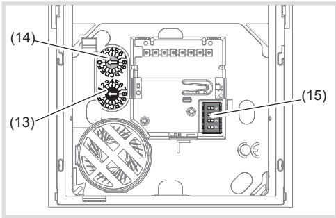
Bild 4: Rückansicht der Bedieneinheit (13) Adressier-Dreheschalter (schwarz) für Gruppenadresse (14) Adressier-Dreheschalter (blau) für Teilnehmeradresse (15) DIP-Schalter für Betriebsarten
