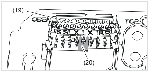
Bild 8: Anschluss-Klemmblock
