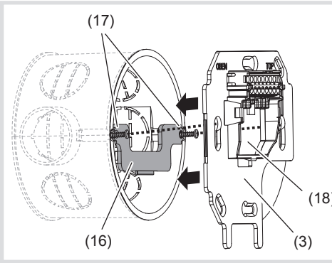
Bild 6: Montage auf Gerätedose
