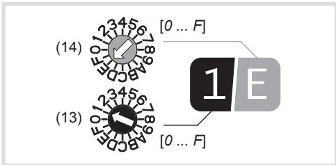
Bild 5: Beispieladresse „1/E“ • Am schwarzen Dreheschalter (13) die Gruppenadresse [0 ... F] einstellen. • Am blauen Dreheschalter (14) die Teilnehmeradresse [0 ... F] einstellen.
