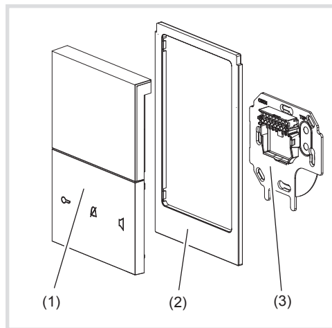
Bild 1: Geräteaufbau
